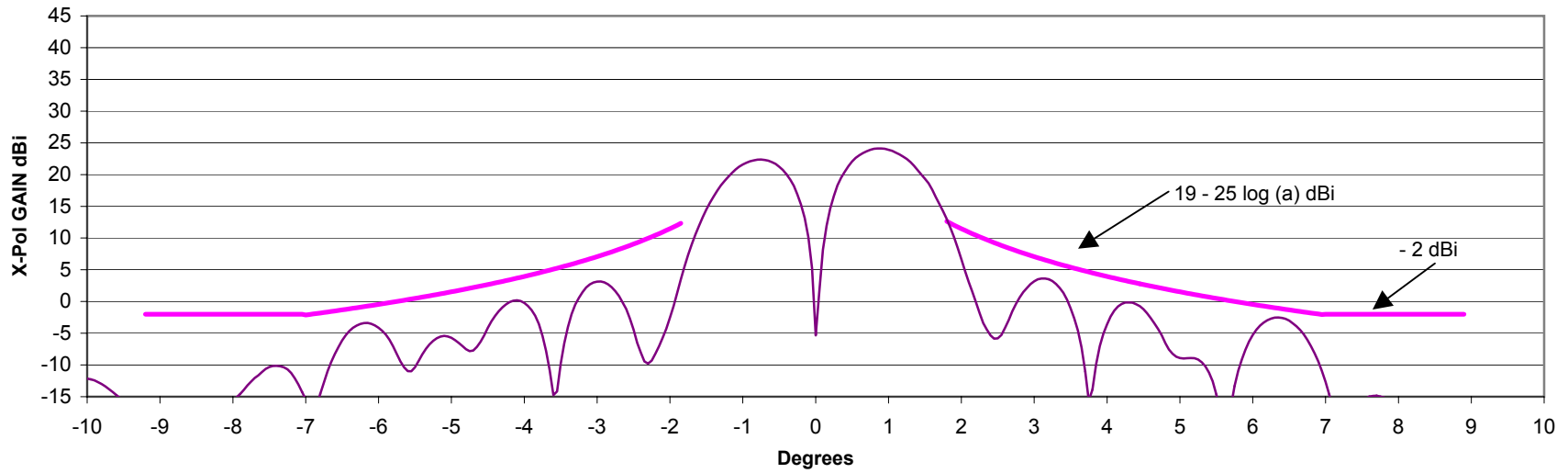
6.04 GHz Cross Pol Gain, Az H-Plane
