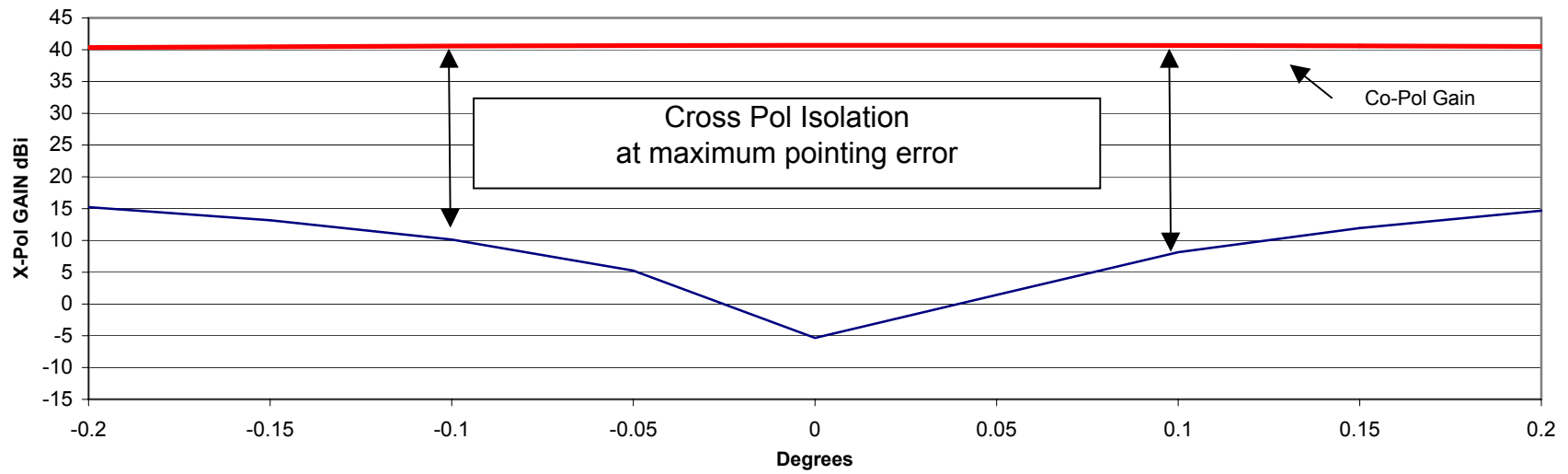
6.04 GHz Cross Pol Isolation, Az H-Plane
