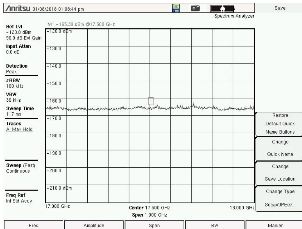
Figure 3.1-3 (D) Spectrum Photos 17-18 GHz 100 kHz Res BW Horizontal Pol Worst Case 225° Azimuth
