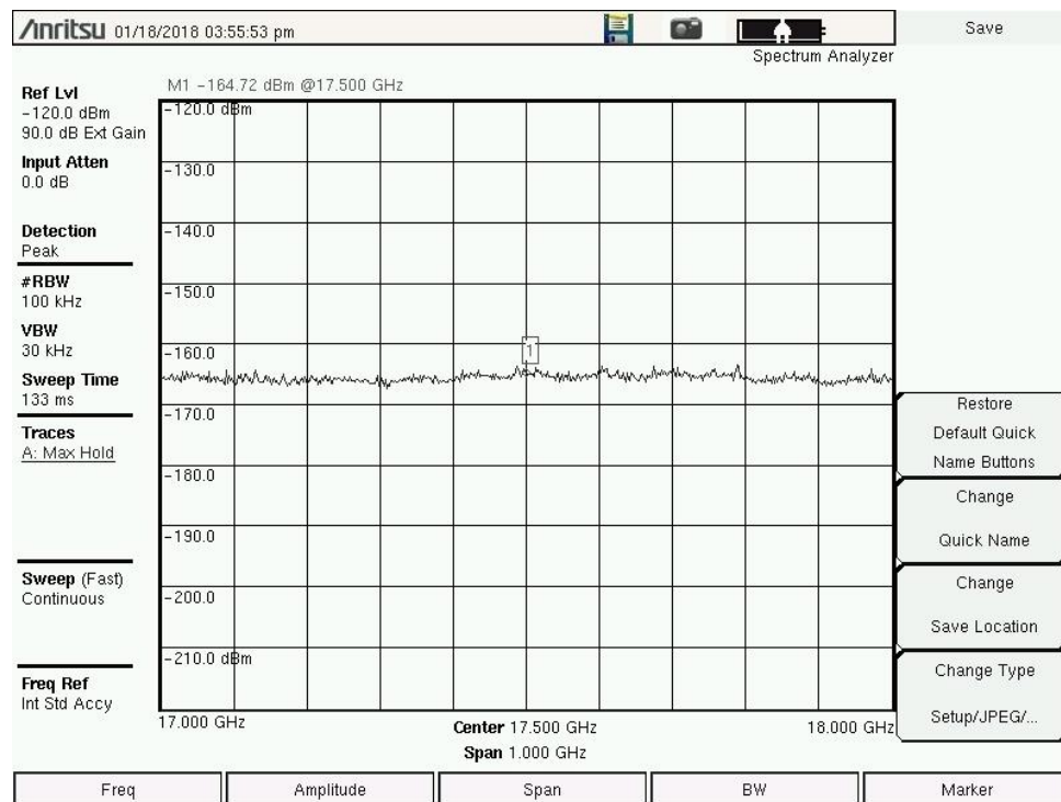
Figure 3.1-3 (D) Spectrum Photos 17-18 GHz 100 kHz Res BW Horizontal Pol Vertical Pol Worst Case 130 degrees 130 degrees
