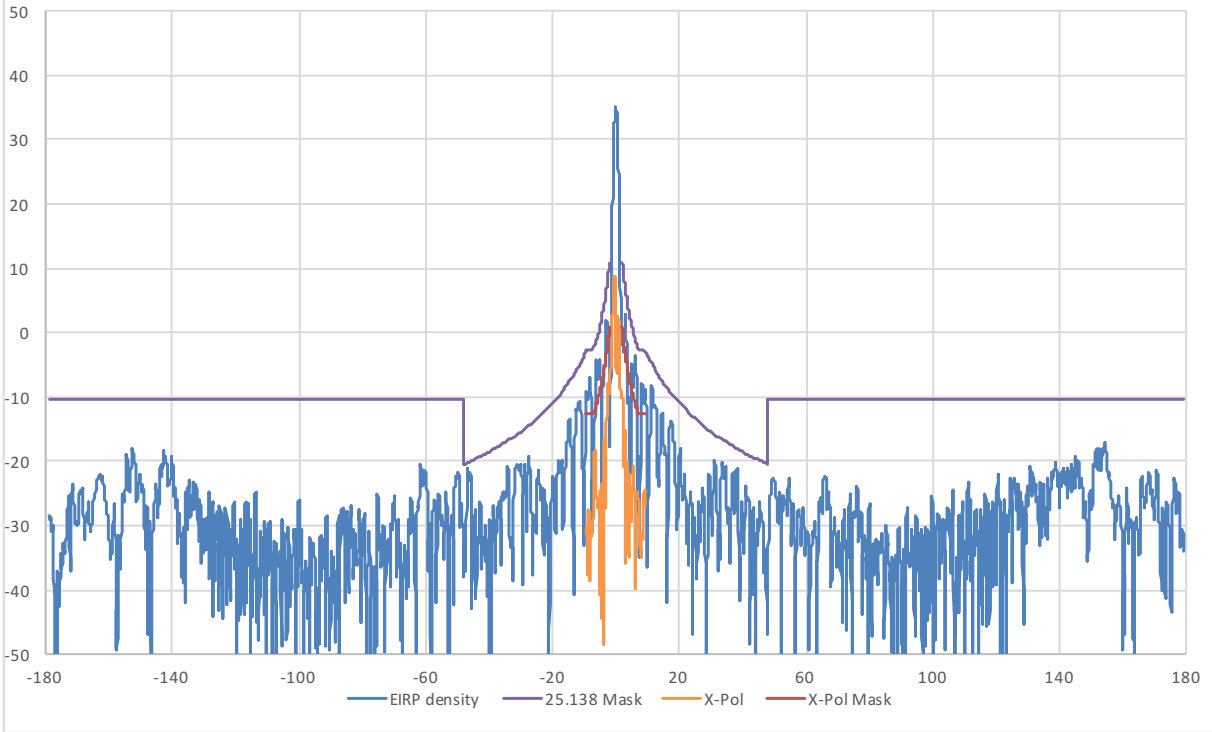
30 GHz Az LHCP EIRP Density Plots
