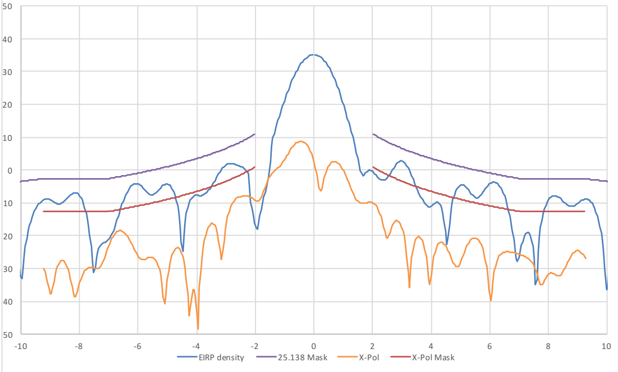
30 GHz Az EIRP Density Plots
