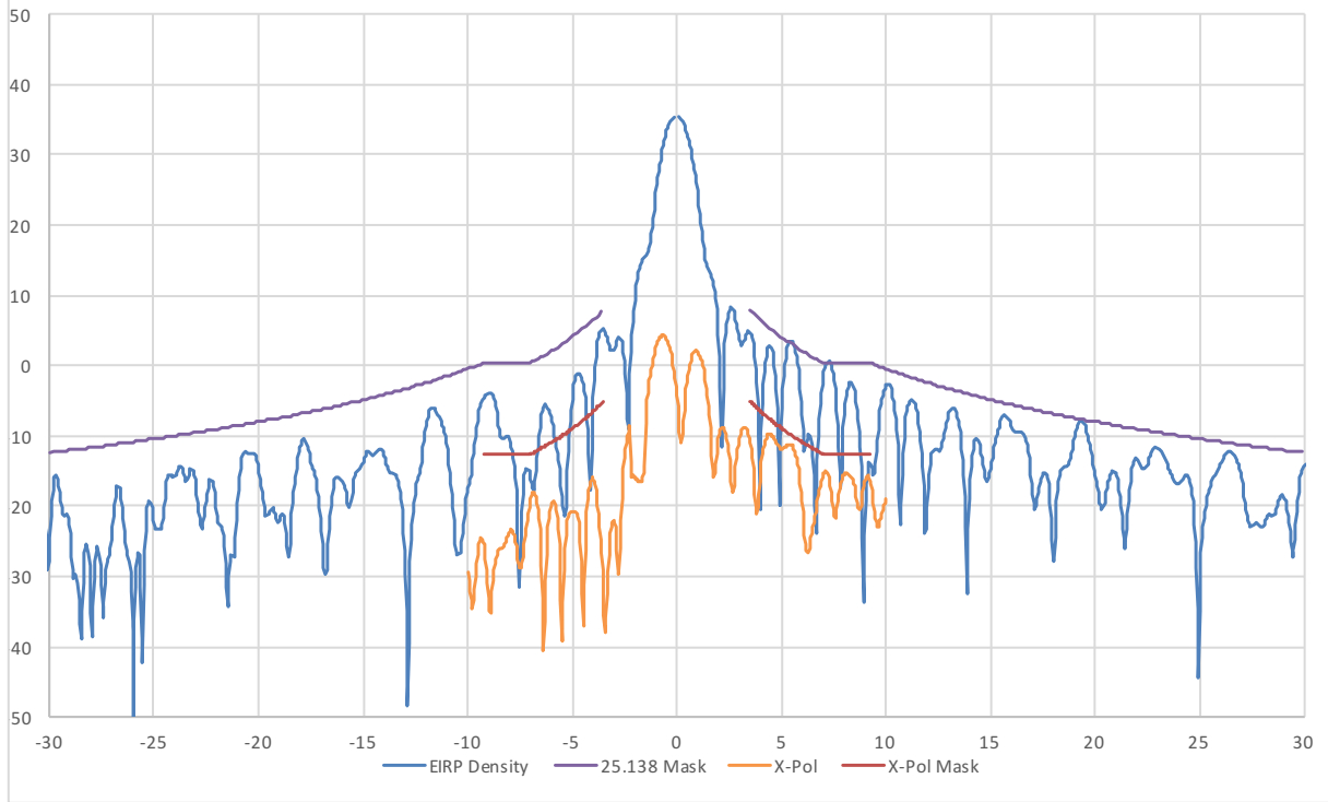
30 GHz EI RHCP EIRP Density Plots
