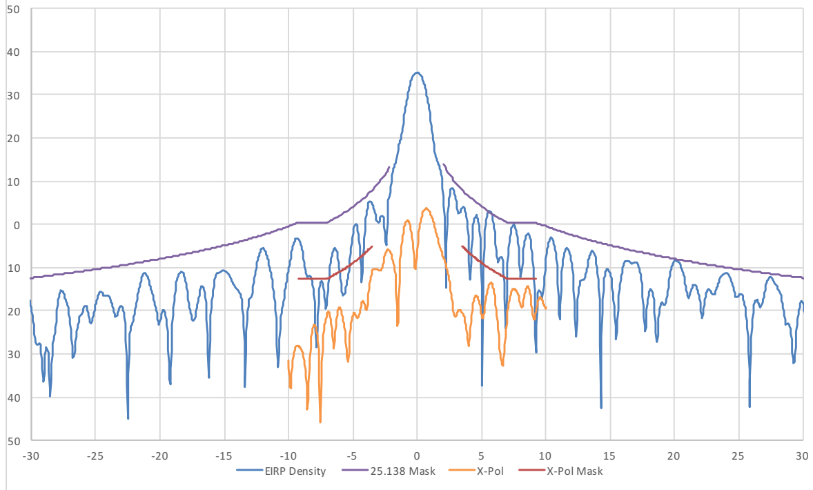
29.1 GHz EI LHCP EIRP Density Plots
