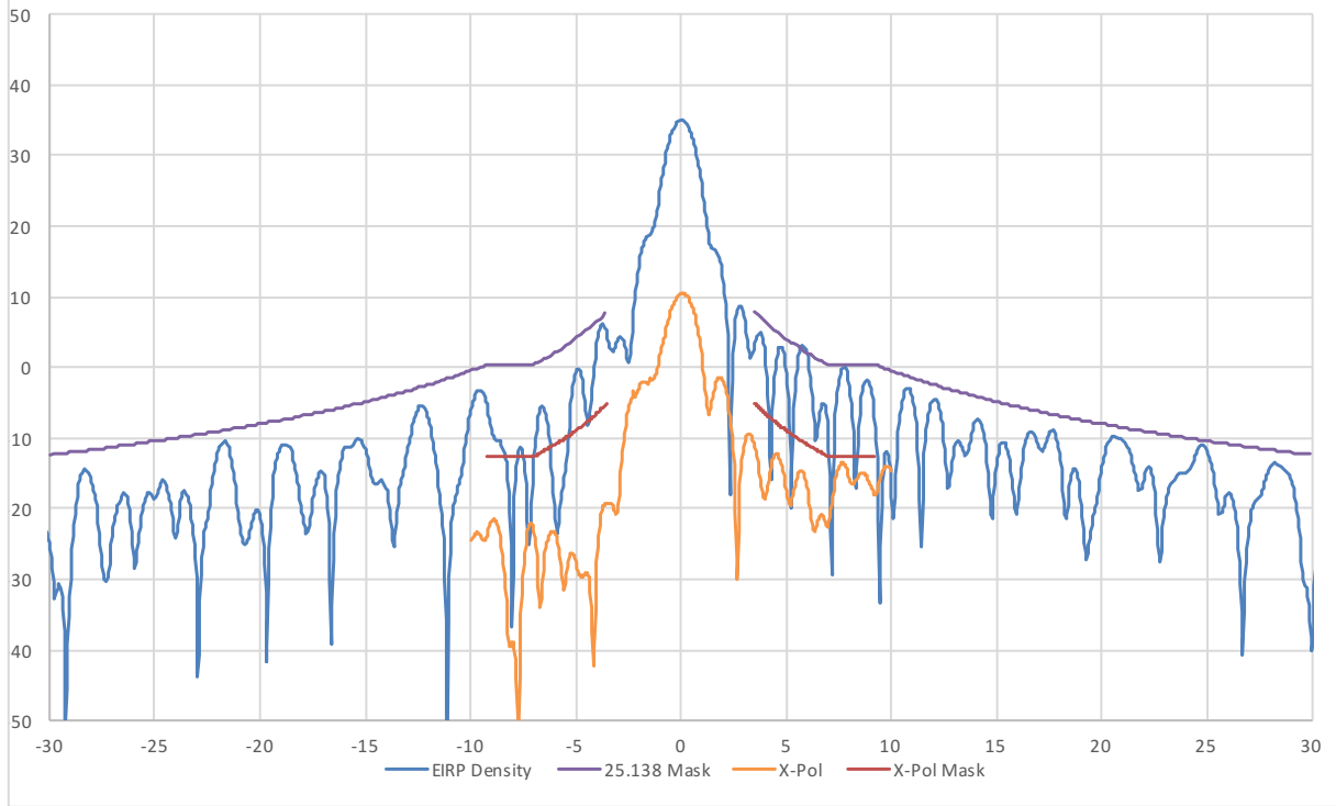
28.35 GHz EI RHCP EIRP Density Plots
