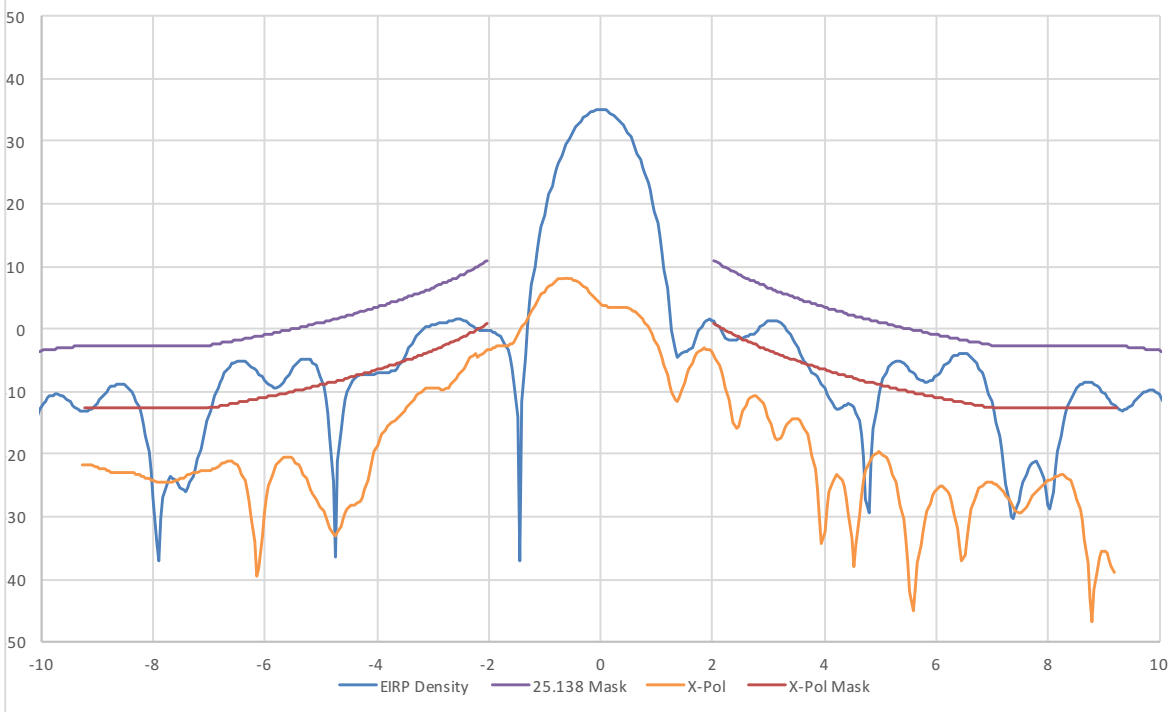
28.35 GHz Az EIRP Density Plots
