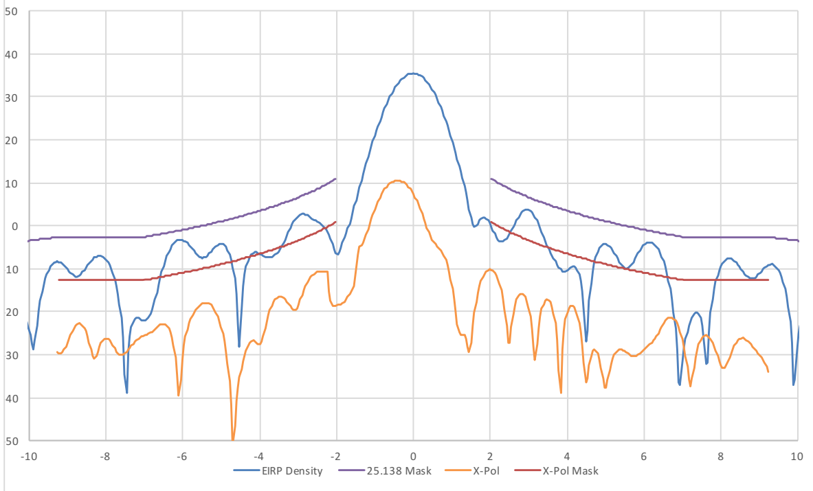
30 GHz Az EIRP Density Plots
