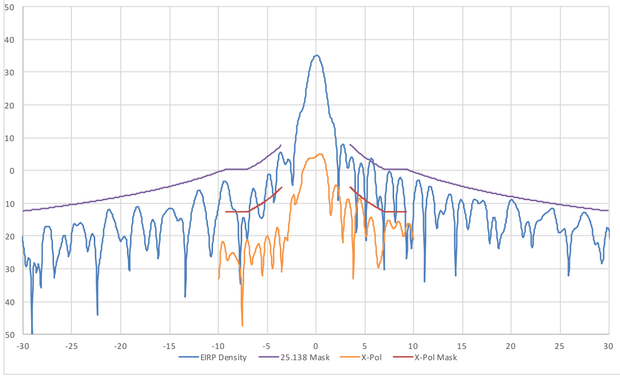
29.1 GHz EI RHCP EIRP Density Plots
