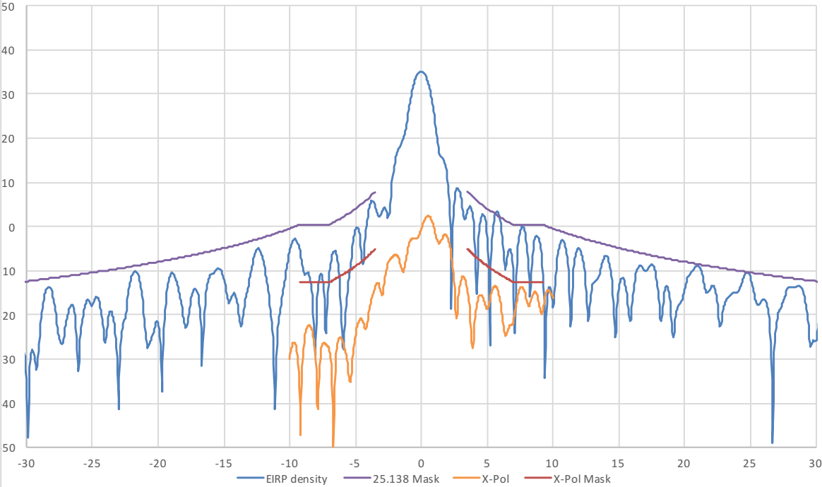
28.35 GHz EI LHCP EIRP Density Plots
