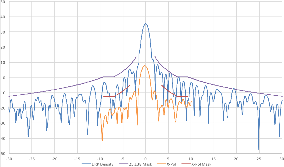
30 GHz EI LHCP EIRP Density Plots
