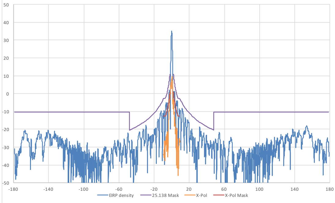
28.35 GHz Az LHCP EIRP Density Plots
