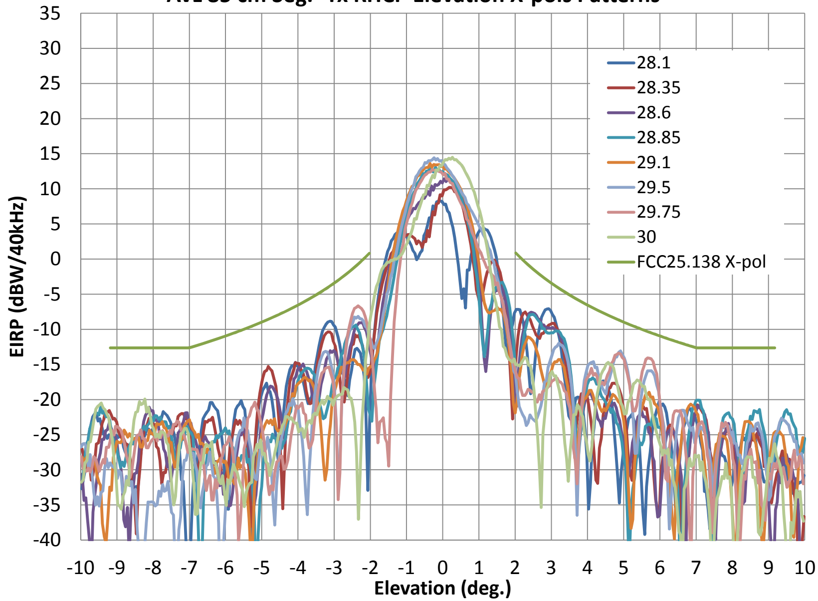
AvL 85 cm Seg.- Tx RHCP Elevation X-pols Patterns
