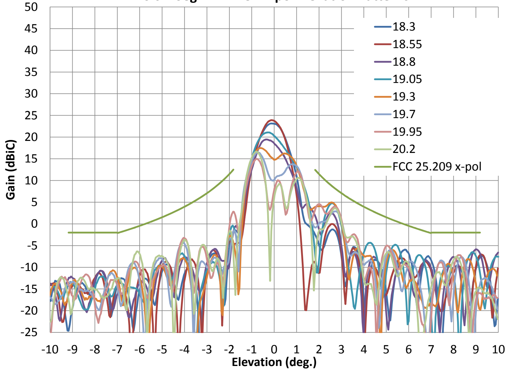
AvL 120 cm Seg.- Rx LHCP X-pol Elevation Patterns
