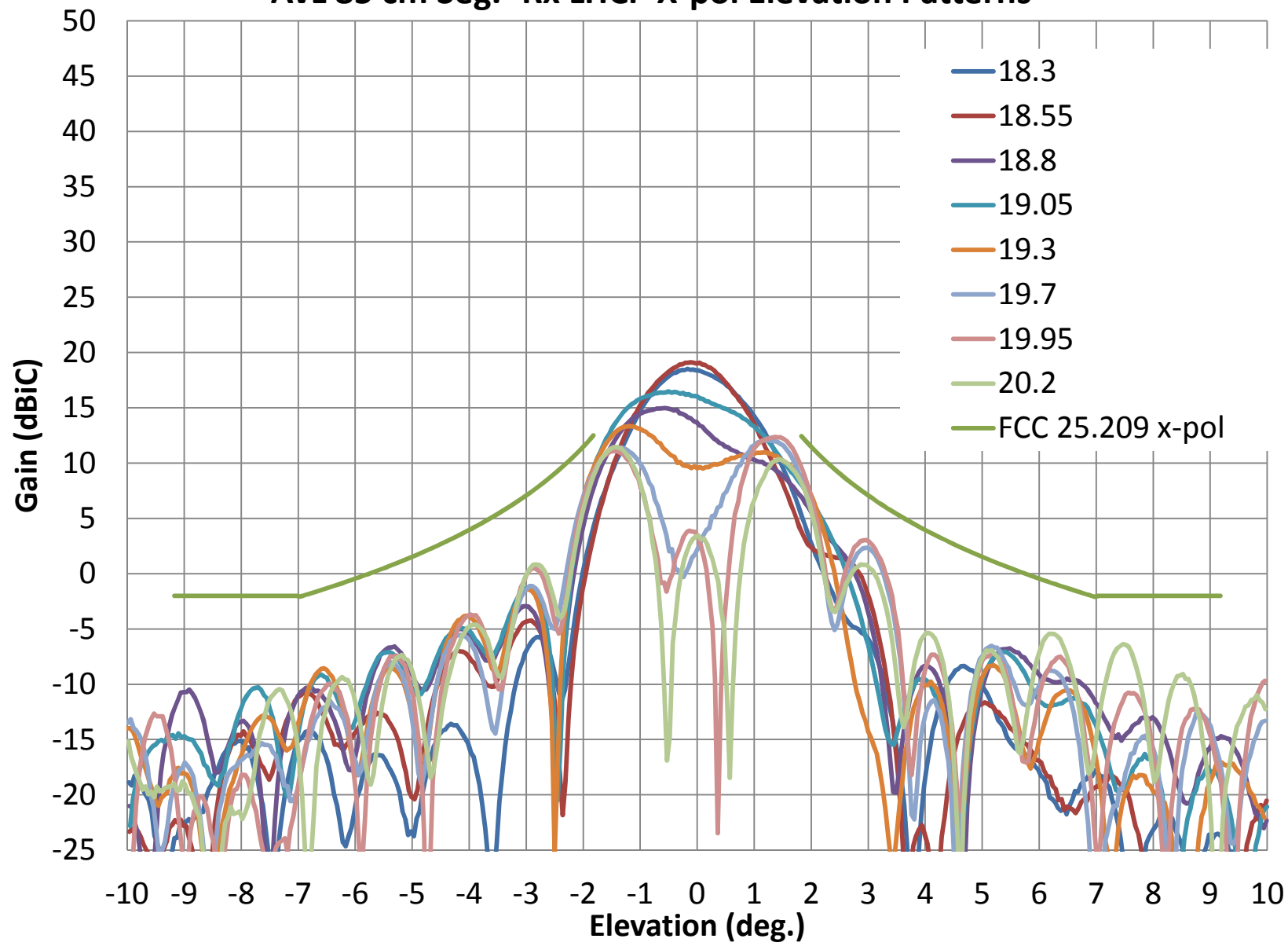
AvL 85 cm Seg.- Rx LHCP X-pol Elevation Patterns
