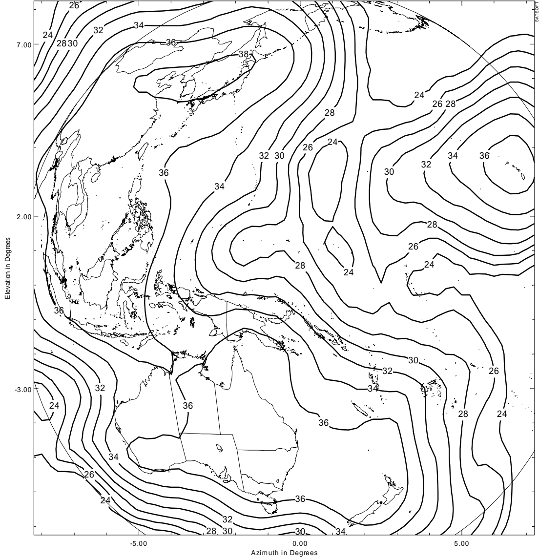
JCSAT-2A C-band Vertical EIRP (dBW)
