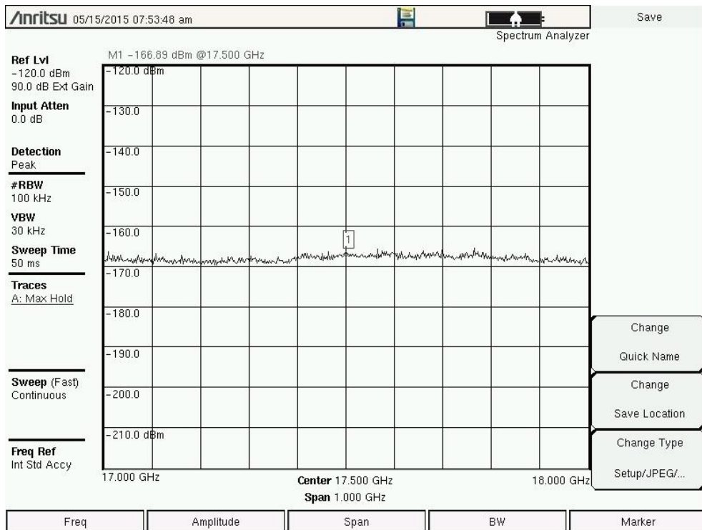
Figure 3.1-3 (D) Spectrum Photos 17-18 GHz 100 kHz Res BW Horizontal Pol Worst
