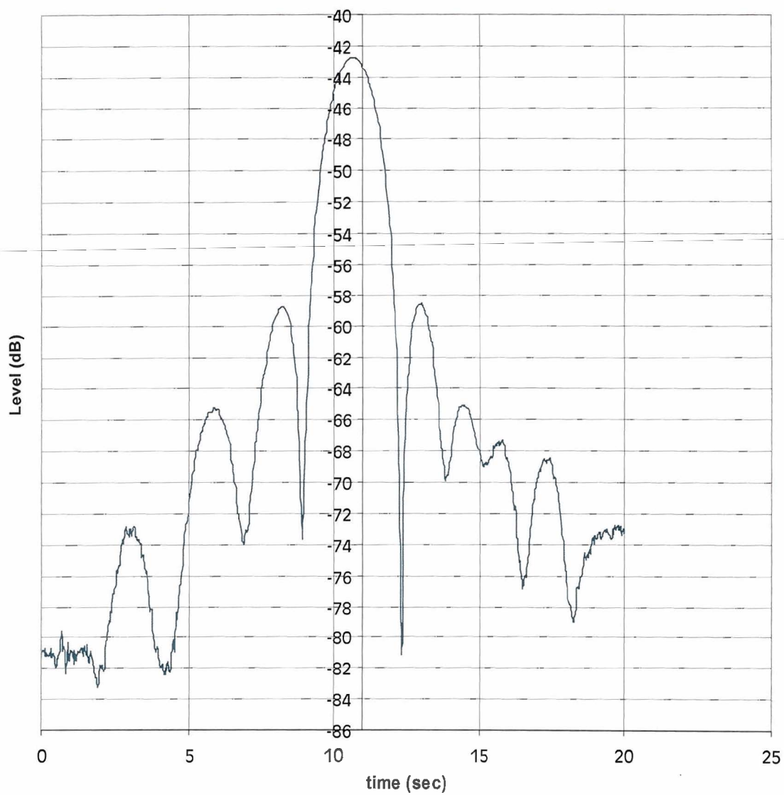
Final AZ pattern
