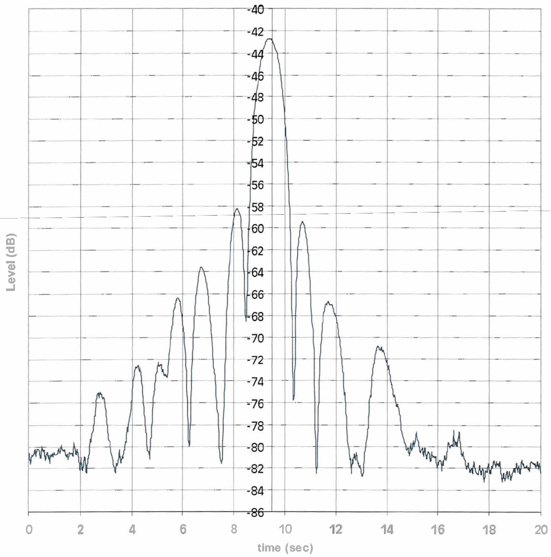
Final EL pattern
