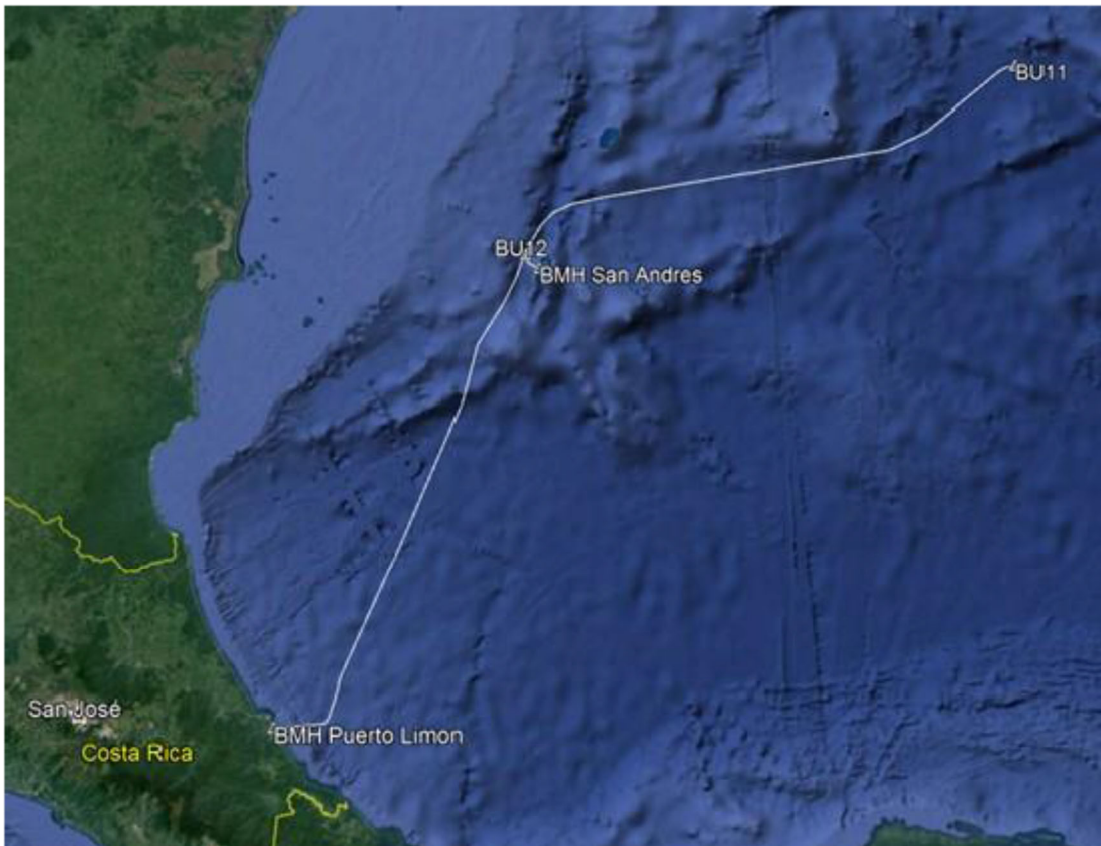
Diagram 2 – Isla San Andrés - Puerto Limón Segment
