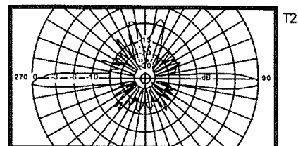
E-Plane
