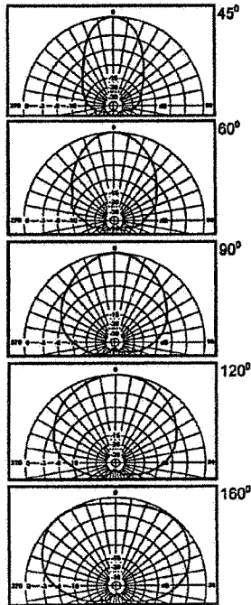
H-Plane
