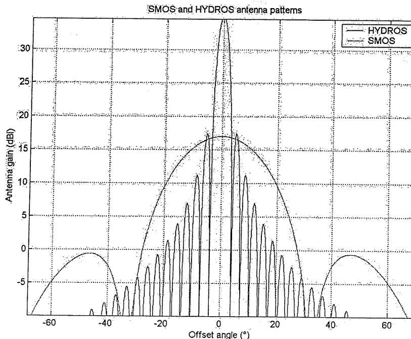
EESS satellites antenna pattern
