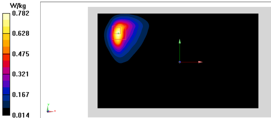
Fig.16 LTE Band5
