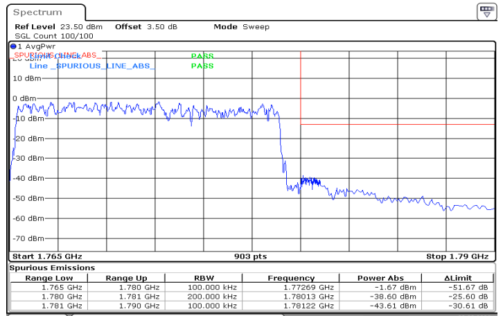
DC_12A_n66A_10MHz|15MHz_15kHz_707.5MHz|1772.5MHz_ DFT-s-OFDM QPSK_RB0|RB75@0
