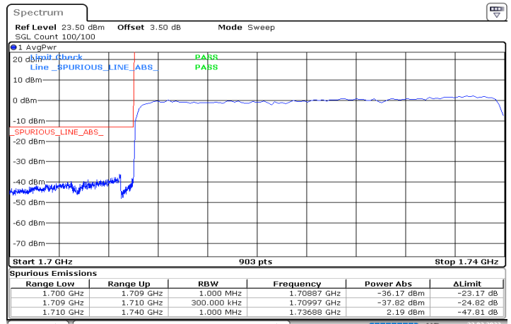
DC_12A_n66A_10MHz|30MHz_15kHz_707.5MHz|1725MHz_ DFT-s-OFDM QPSK_RB0|RB160@0
