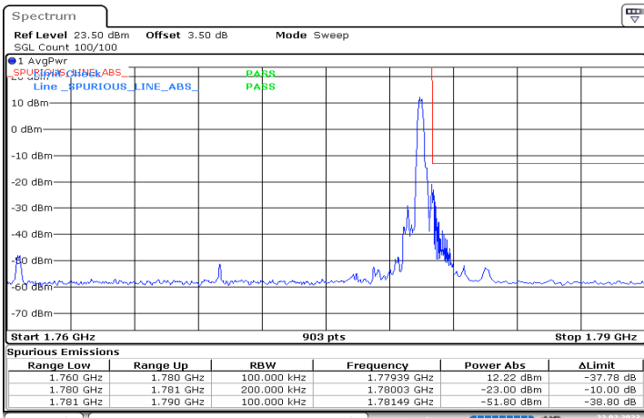
DC_12A_n66A_10MHz|20MHz_15kHz_707.5MHz|1770MHz_ DFT-s-OFDM QPSK_RB0|RB1@105
