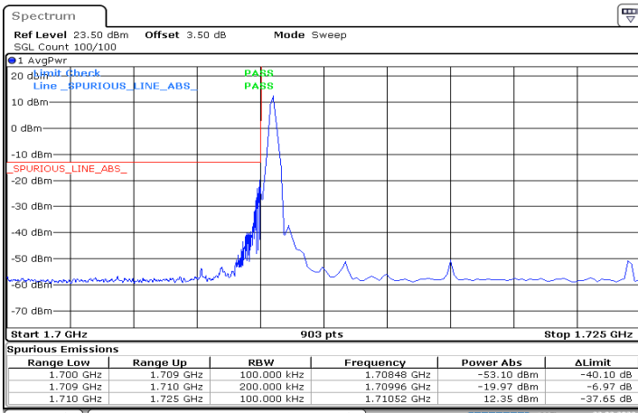
DC_12A_n66A_10MHz|15MHz_15kHz_707.5MHz|1717.5MHz_ DFT-s-OFDM QPSK_RB0|RB1@0
