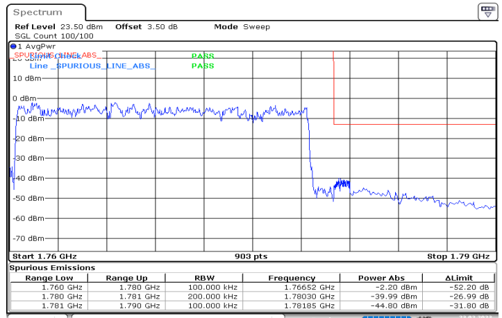
DC_12A_n66A_10MHz|20MHz_15kHz_707.5MHz|1770MHz_ DFT-s-OFDM QPSK_RB0|RB100@0
