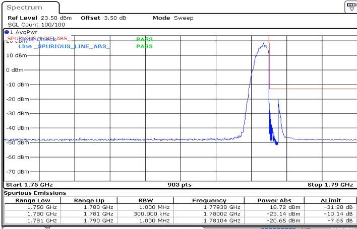
DC_12A_n66A_10MHz|30MHz_15kHz_707.5MHz|1765MHz_ DFT-s-OFDM QPSK_RB0|RB1@159
