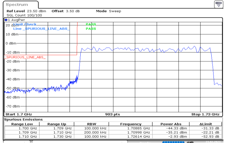
DC_12A_n66A_10MHz|20MHz_15kHz_707.5MHz|1720MHz_ DFT-s-OFDM QPSK_RB0|RB100@0
