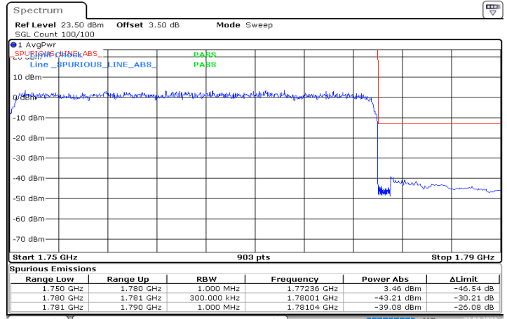
DC_12A_n66A_10MHz|30MHz_15kHz_707.5MHz|1765MHz_ DFT-s-OFDM QPSK_RB0|RB160@0
