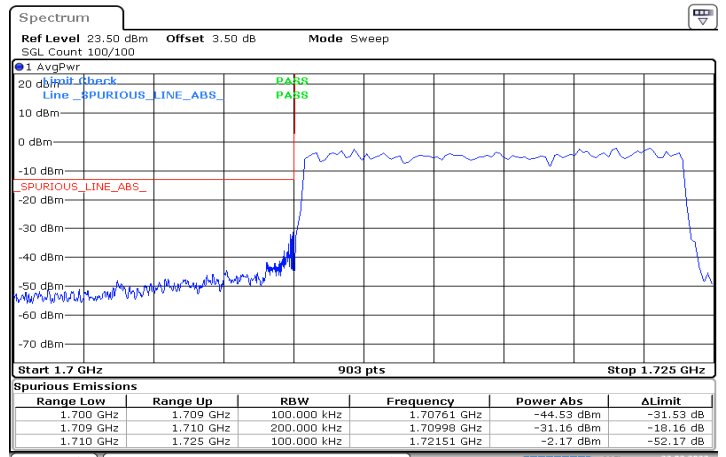
DC_12A_n66A_10MHz|15MHz_15kHz_707.5MHz|1717.5MHz_ DFT-s-OFDM QPSK_RB0|RB75@0
