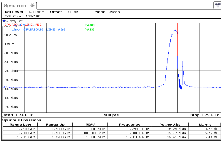
DC_12A_n66A_10MHz|40MHz_15kHz_707.5MHz|1760MHz_ DFT-s-OFDM QPSK_RB0|RB1@215
