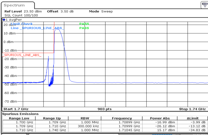
DC_12A_n66A_10MHz|30MHz_15kHz_707.5MHz|1725MHz_ DFT-s-OFDM QPSK_RB0|RB1@0
