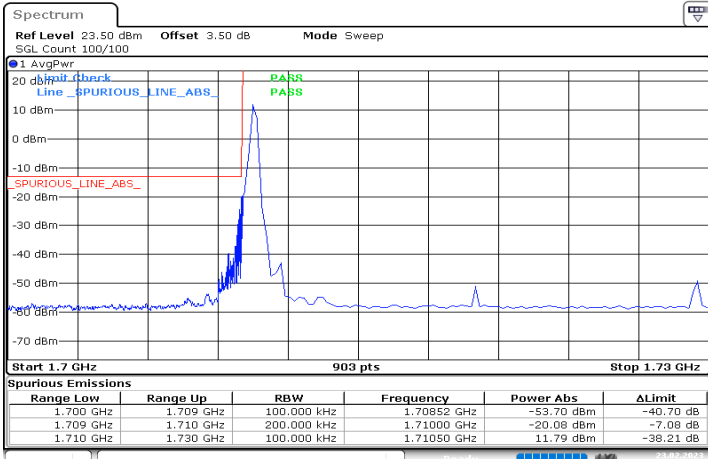
DC_12A_n66A_10MHz|20MHz_15kHz_707.5MHz|1720MHz_ DFT-s-OFDM QPSK_RB0|RB1@0
