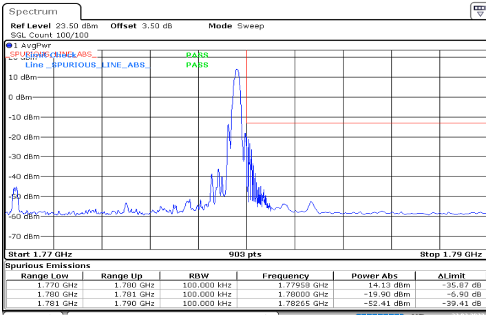
DC_12A_n66A_10MHz|10MHz_15kHz_707.5MHz|1775MHz_ DFT-s-OFDM QPSK_RB0|RB1@51
