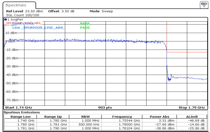
DC_12A_n66A_10MHz|40MHz_15kHz_707.5MHz|1760MHz_ DFT-s-OFDM QPSK_RB0|RB216@0
