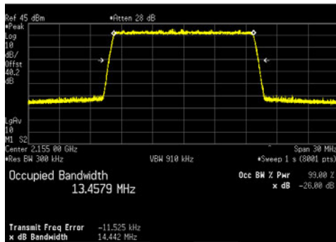
LTE15_QPSK
