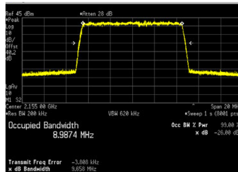
LTE10_16QAM
