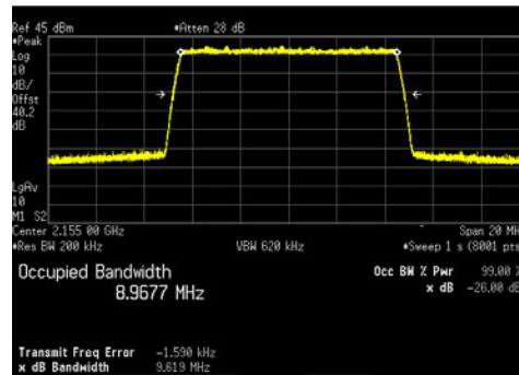
LTE10_QPSK
