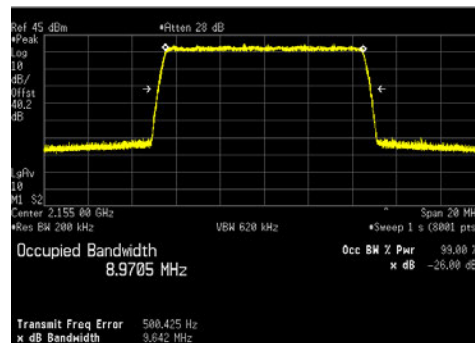
LTE10_64QAM
