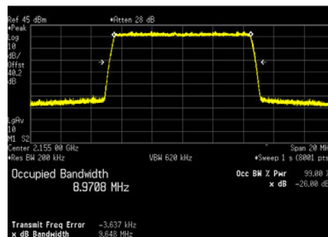
LTE10_256QAM
