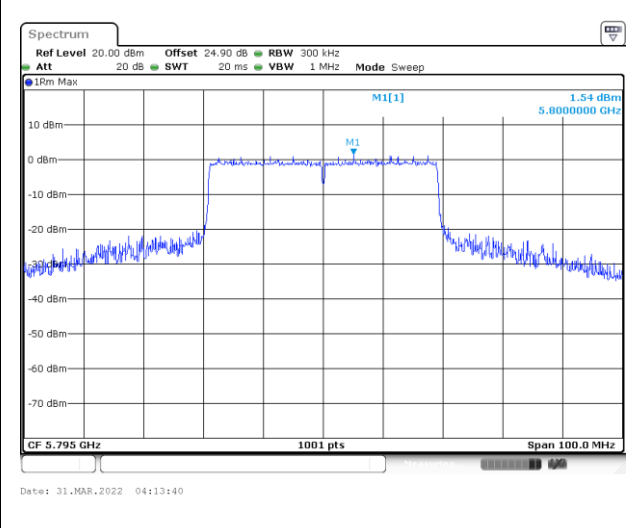
MIMO Ant. 8
