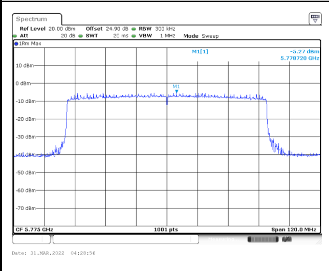
MIMO Ant. 9
