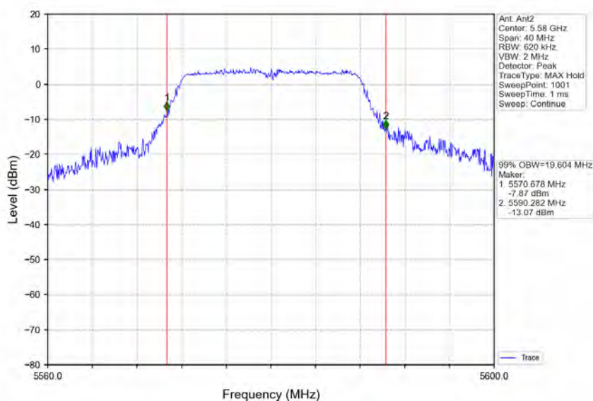
802.11a MCH 5580MHz Ant2 NTNv
