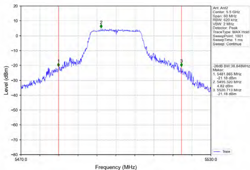
802.11a LCH_5500MHz_Ant2_NTNV
