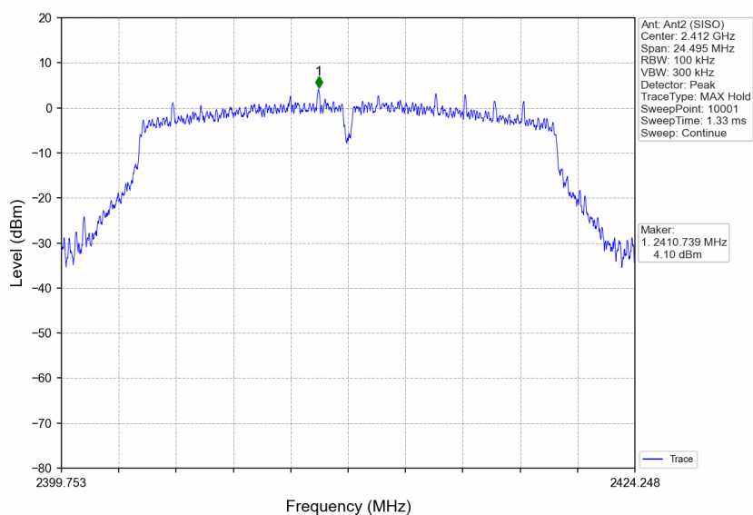
802.11n(HT20)_LCH_2412MHz_Ant2 (SISO)_NTNV
