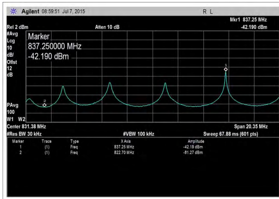
UL_824-849MHz-AWGNR+1
