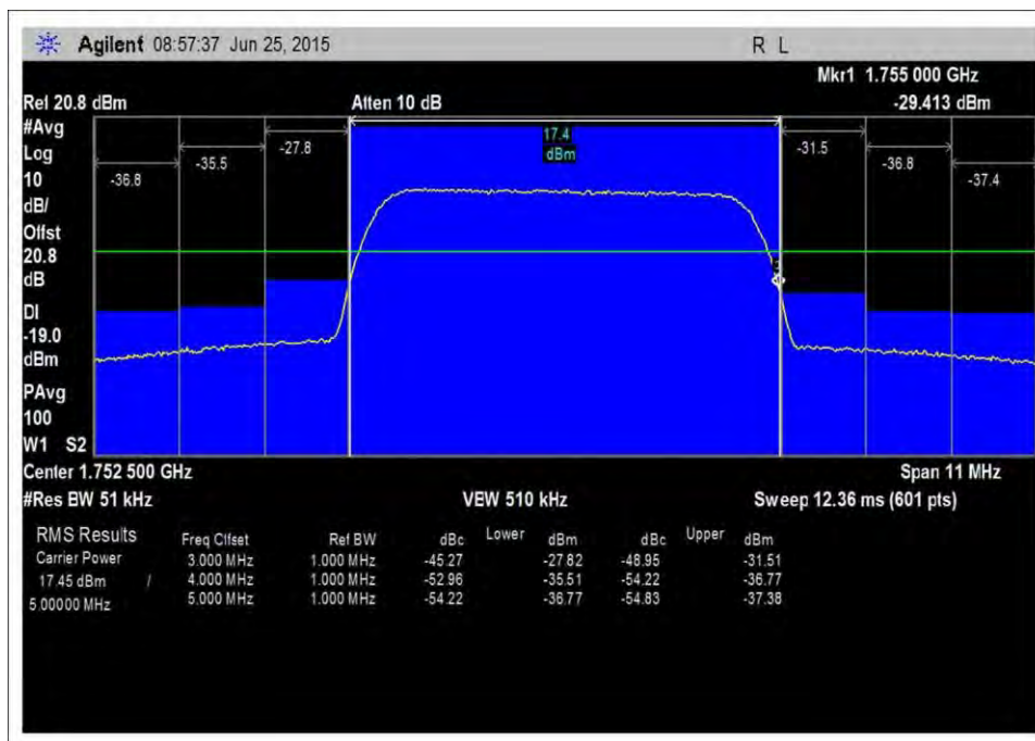
UL_1710-1755MHz_H_PreAGC
