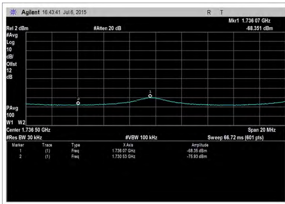
UL_1710-1755MHz-AWGNL+3
