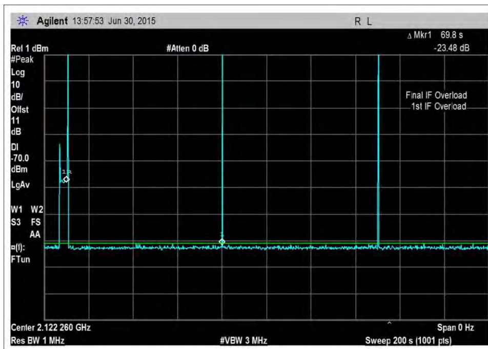
DL_2110-2155MHz-200sec
