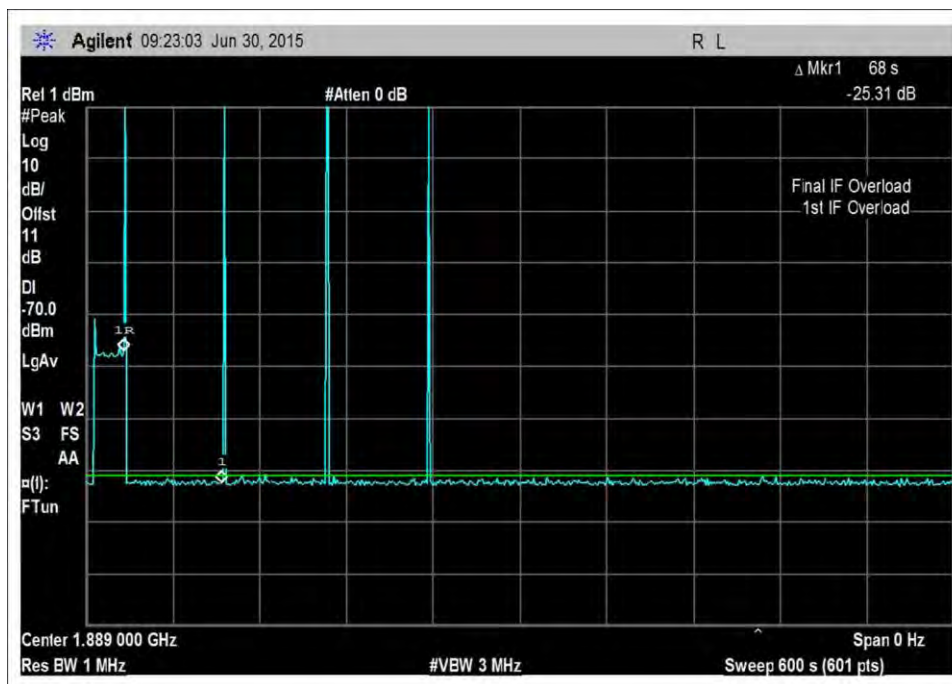
UL_1850-1915MHz-600sec
