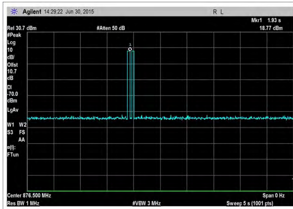
DL_869-894MHz-Pk
