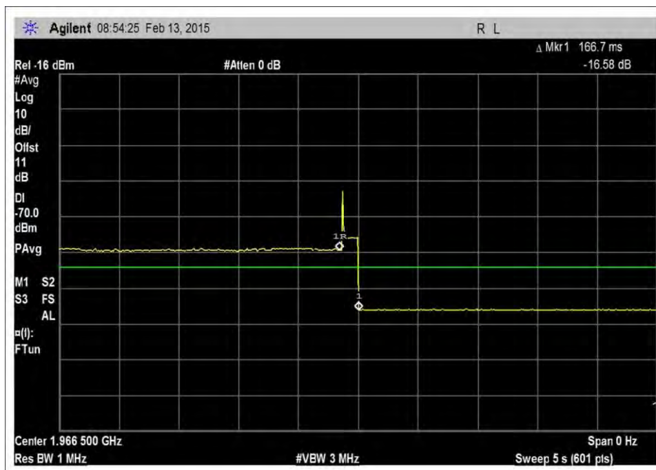
DL_1930-1995MHz_a-g_timing
