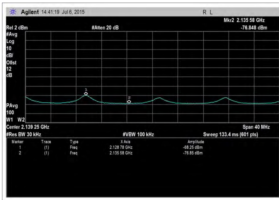
DL_2110-2155MHz-AWGNL+2
