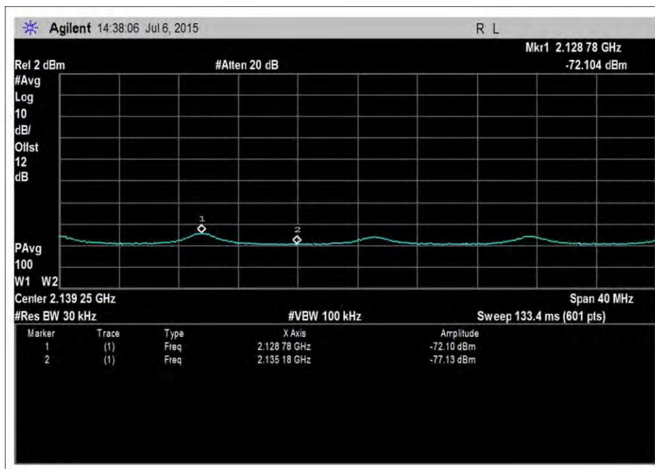
DL_2110-2155MHz-AWGNL+3
