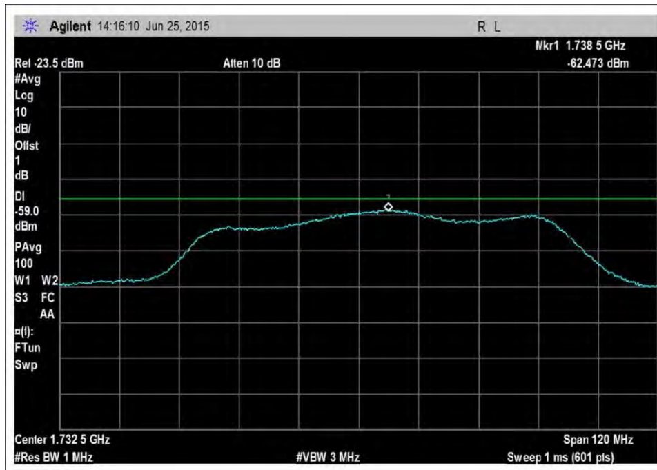
UL_1710-1755MHz-Zoom_a-g_Noise_50
