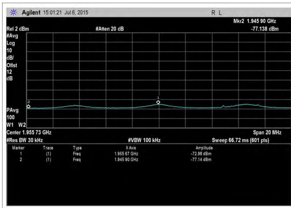
DL_1930-1995MHz-AWGNL+3
