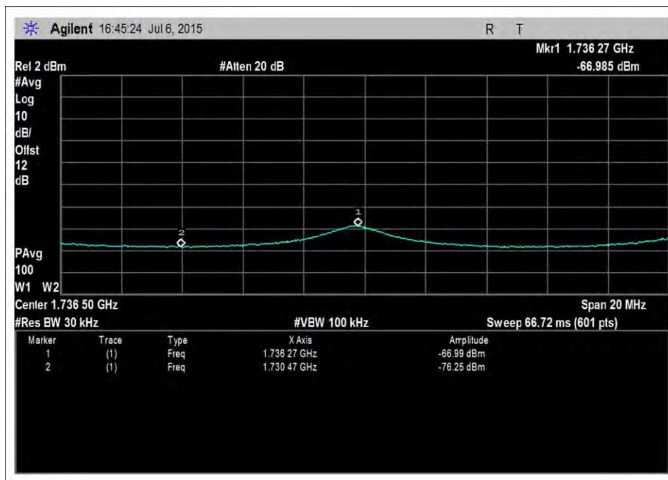
UL_1710-1755MHz-AWGNL+2
