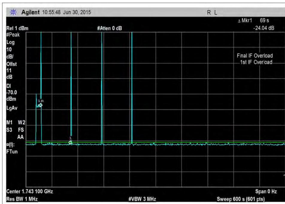
UL_1710-1755MHz-600sec
