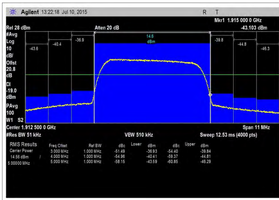
UL_1850-1915MHz_H_PreAGC
