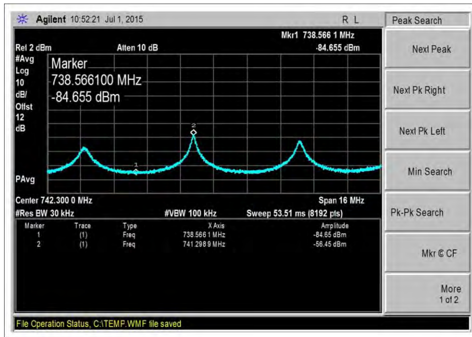
DL_728-746MHz-AWGNL+0
