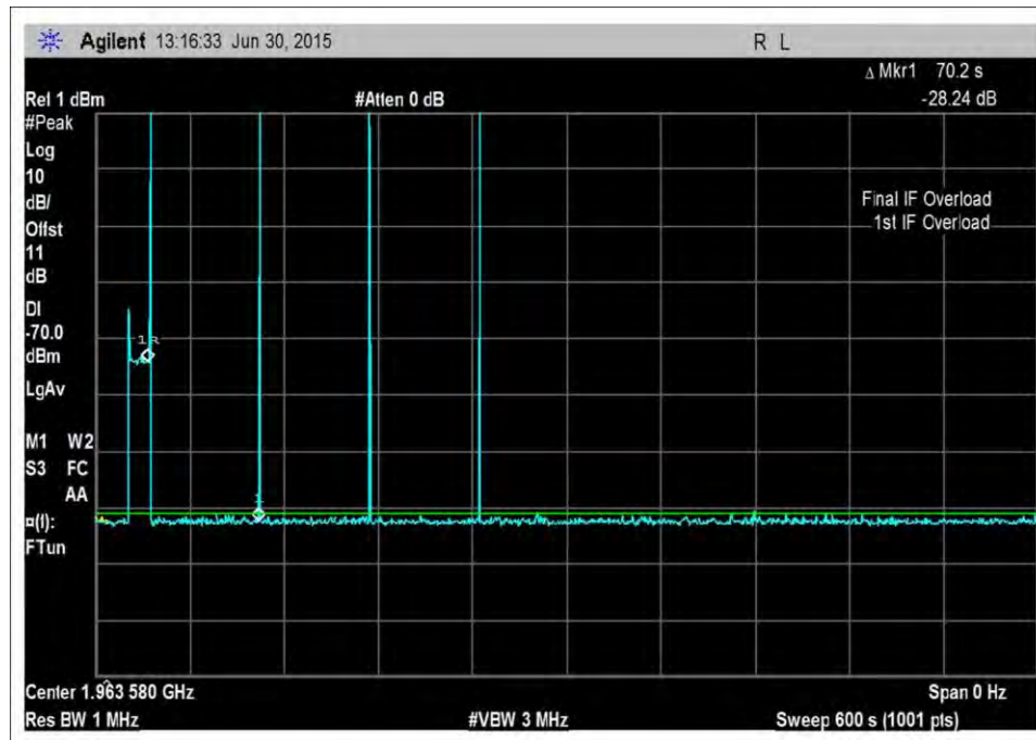
DL_1930-1995MHz-600sec
