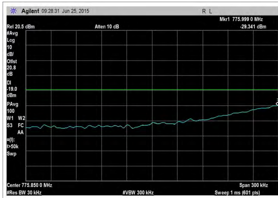
UL_776-787MHz_L_Max
