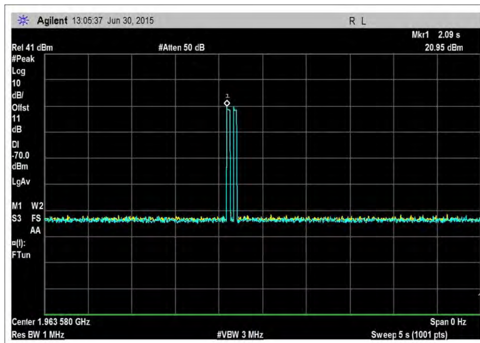
DL_1930-1995MHz-Pk
