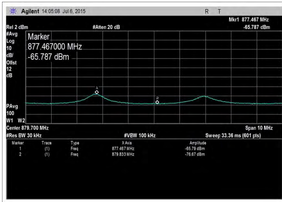
DL_869-894MHz-AWGNL+4
