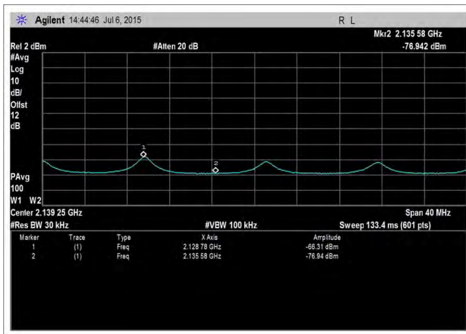
DL_2110-2155MHz-AWGNL+1
