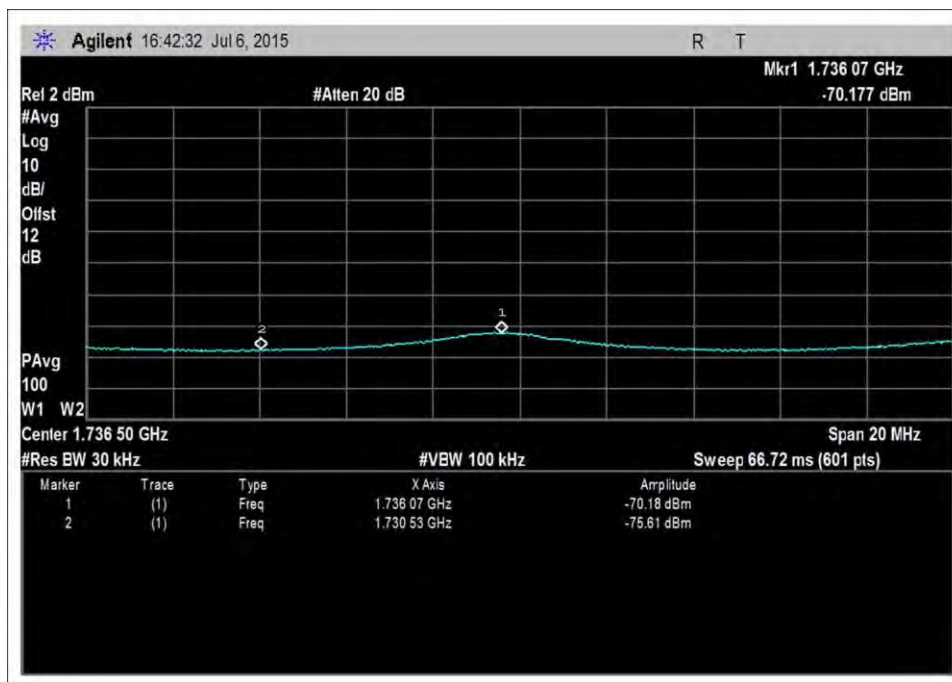
UL_1710-1755MHz-AWGNL+5
