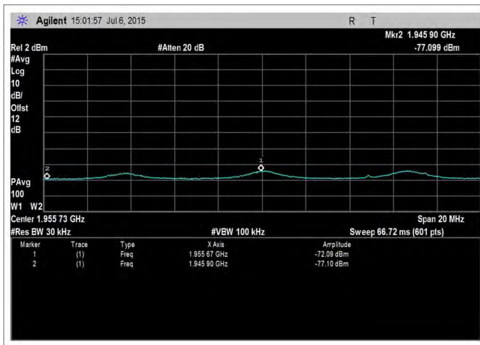
DL_1930-1995MHz-AWGNL+2
