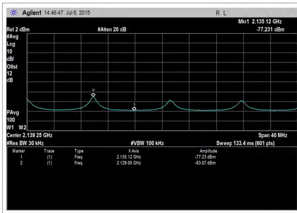
DL_2110-2155MHz-AWGNL+0
