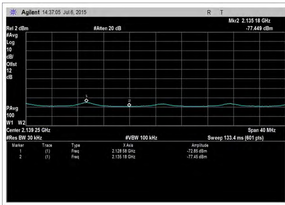
DL_2110-2155MHz-AWGNL+4
