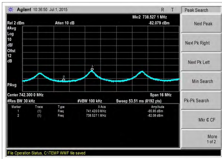
DL_728-746MHz-AWGNL+1
