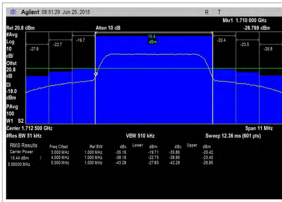
UL_1710-1755MHz_L_PreAGC
