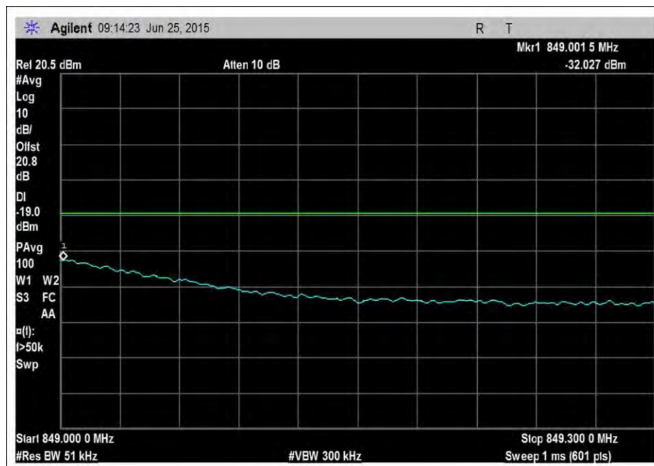
UL_824-849MHz_H_PreAGC
