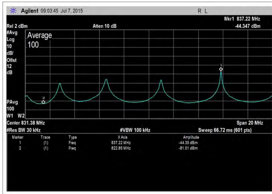
UL_824-849MHz-AWGNR+0
