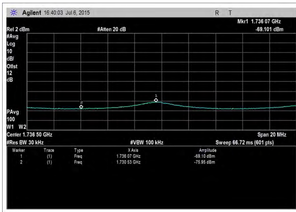
UL_1710-1755MHz-AWGNL+4
