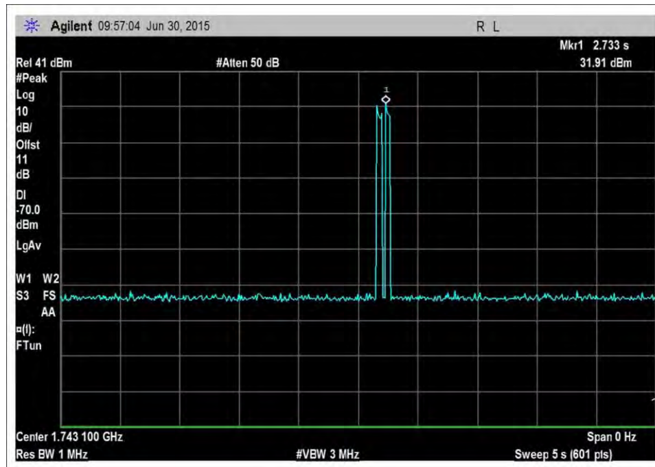
UL_1710-1755MHz-Pk
