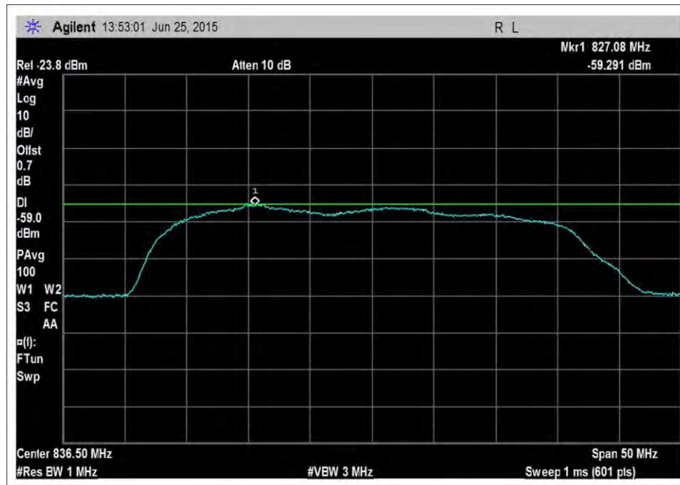
UL_824-849MHz_a-g_Noise_50
