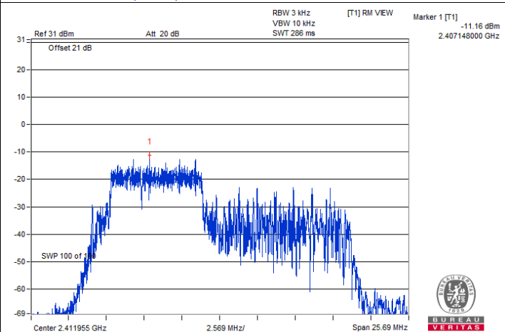
802.11be (EHT 20M) 52+26-tone MRU / Chain 0 : CH 1@70
