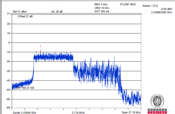
802.11be (EHT) 106-tone RU / Chain 1 : CH 6@53
