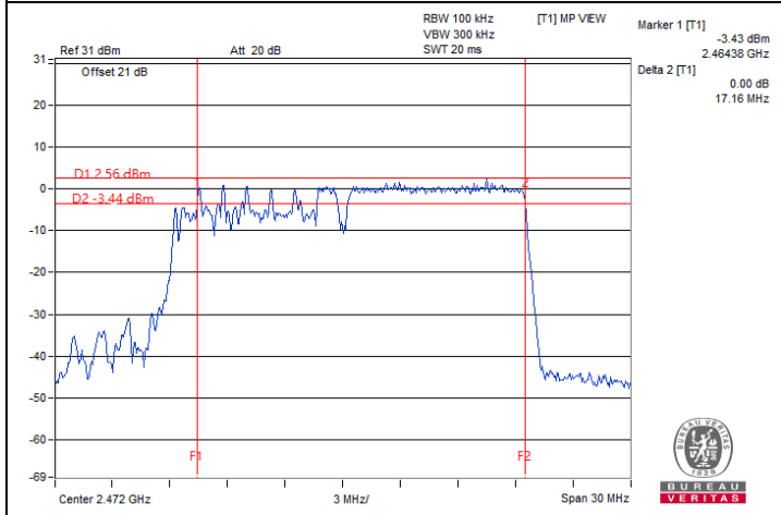
802.11be (EHT 20M) 106+26-tone MRU / Chain 0 : CH 13@83
