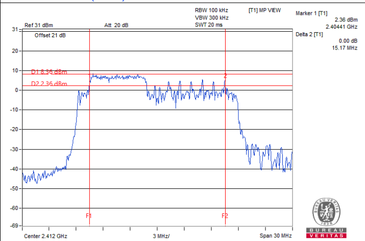
802.11be (EHT 20M) 52+26-tone MRU / Chain 1 : CH 1@70
