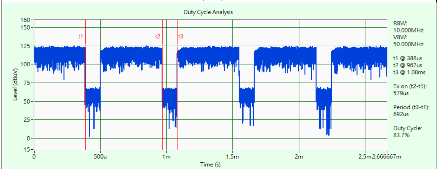
802.11be (EHT 20M) 52+26-tone MRU
