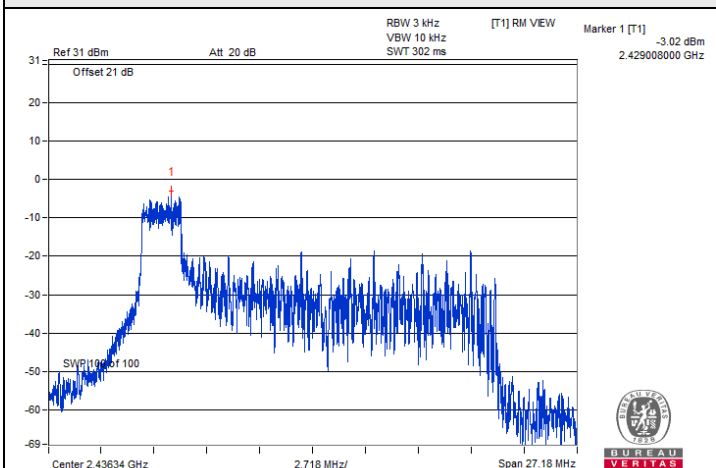
802.11be (EHT) 26-tone RU / Chain 1 : CH 6@0
