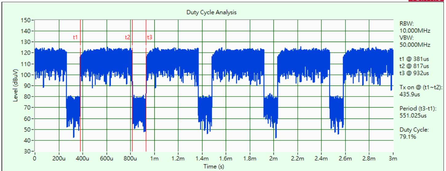
802.11be (EHT) 106-tone RU
