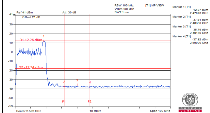
Chain 1 : CH 11@8 Band edge
