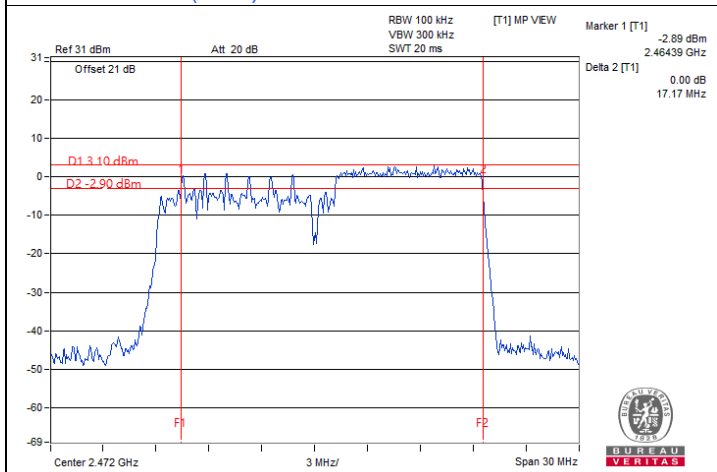
802.11be (EHT) 106-tone RU / Chain 0 : CH 13@54
