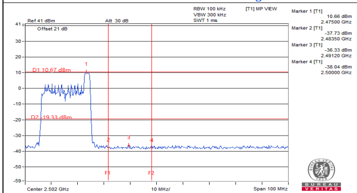
Chain 1 : CH 12@8 Band edge
