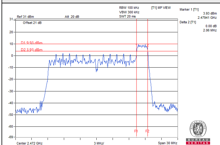
802.11be (EHT) 26-tone RU / Chain 0 : CH 13@8
