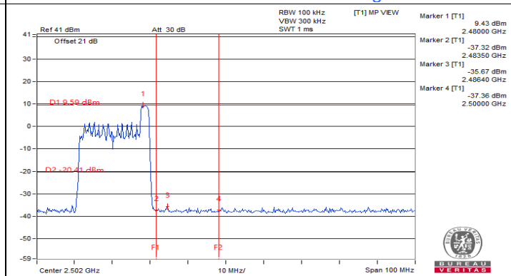
Chain 1 : CH 13@8 Band edge
