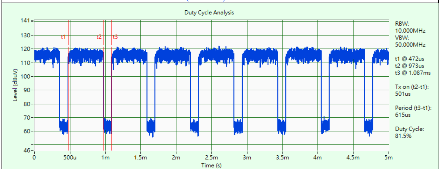
802.11be (EHT 20M) 106+26-tone MRU
