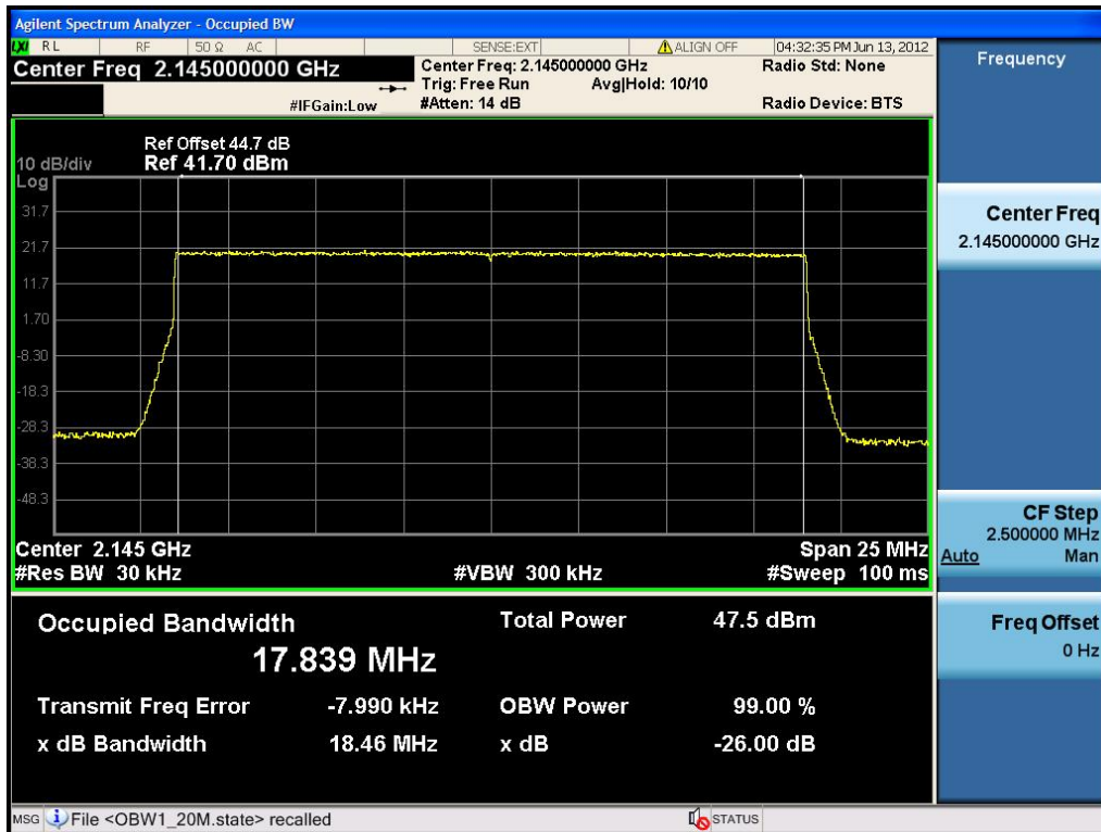
20M-Port 2 -2120MHz
