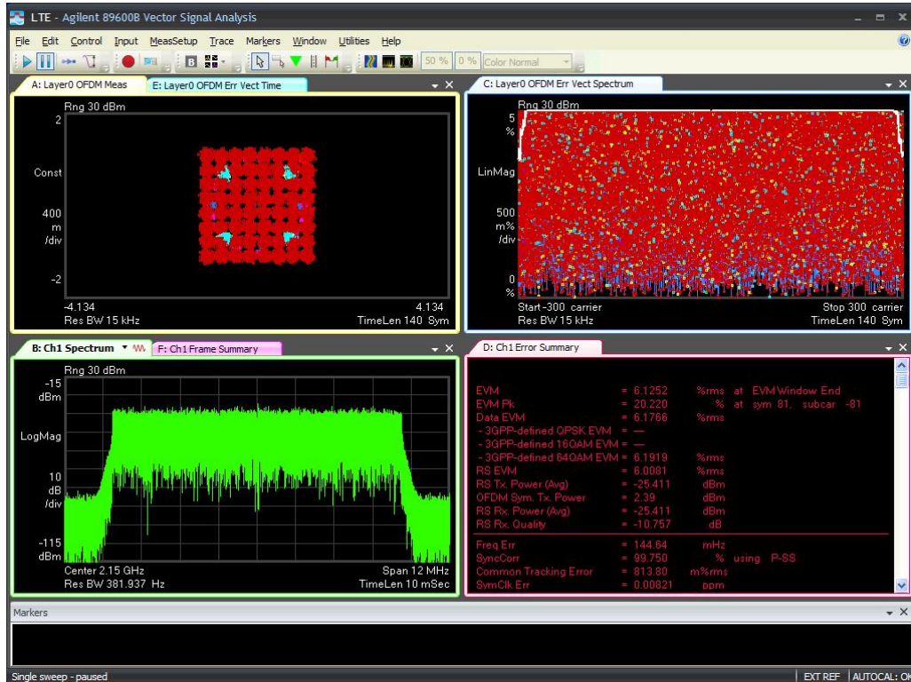
10M-Port 2 -2150MHz-TM3.2
