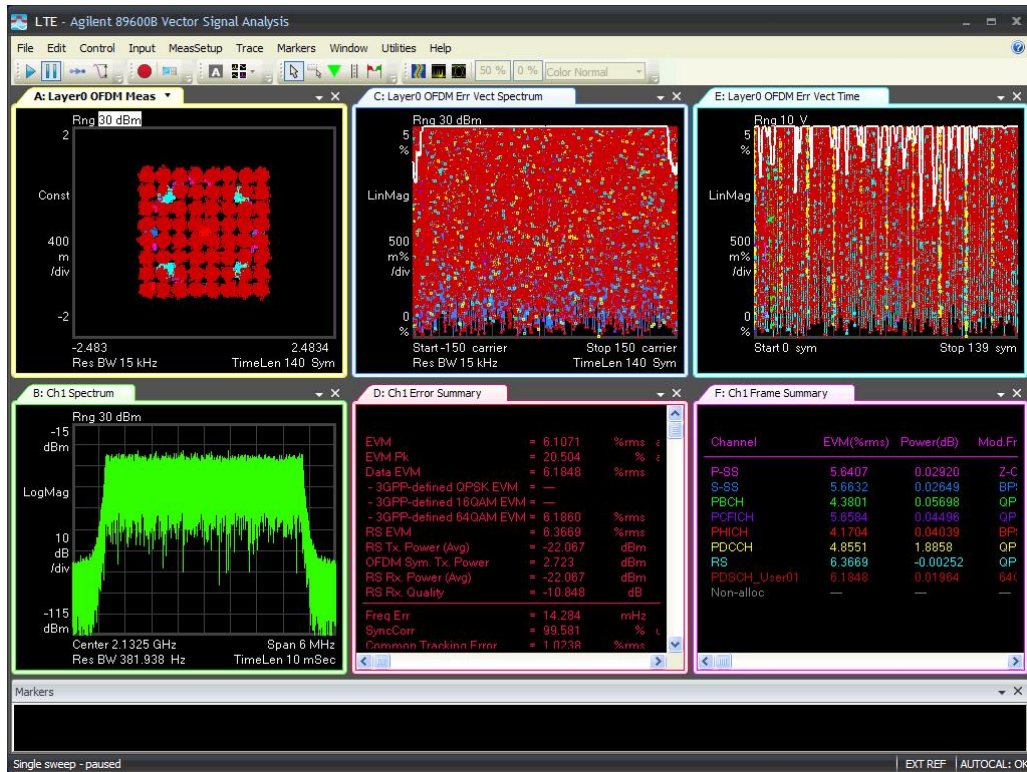
5M-Port 1 -2132.5MHz-TM3.2
