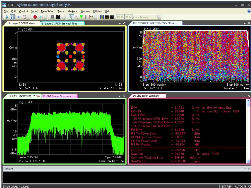
10M-Port 2 -2150MHz-TM2.0
