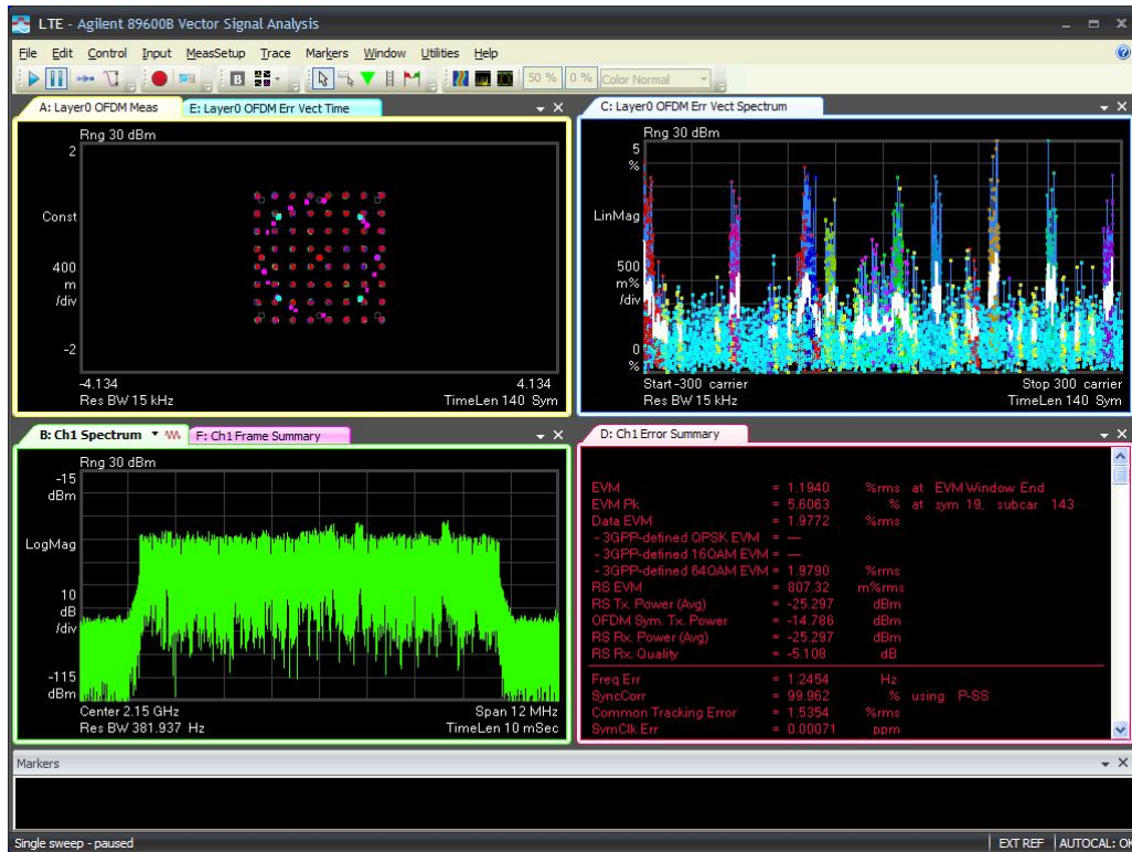
10M-Port 2 -2150MHz-TM3.1
