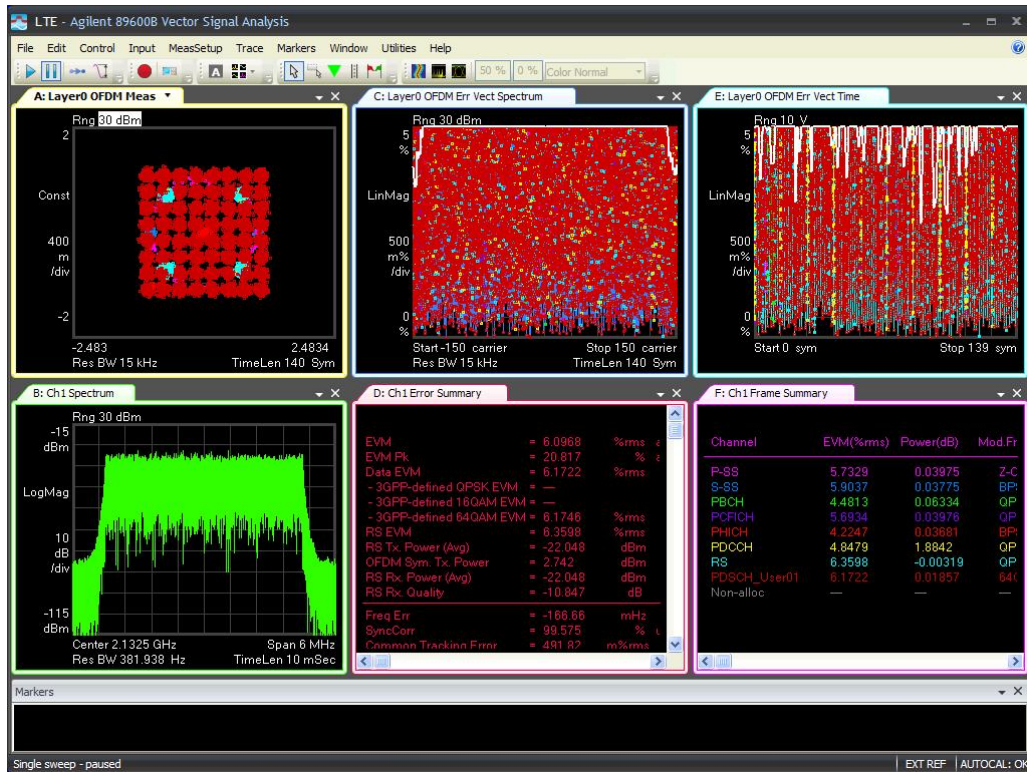
5M-Port 2 -2132.5MHz-TM3.2
