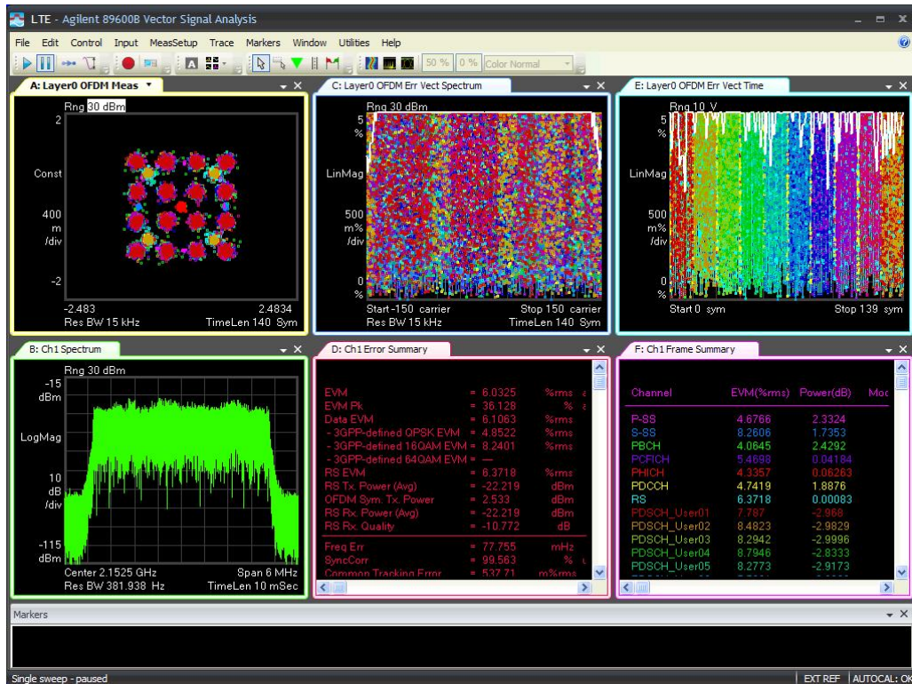
5M-Port 1 - 2152.5MHz-TM3.3
