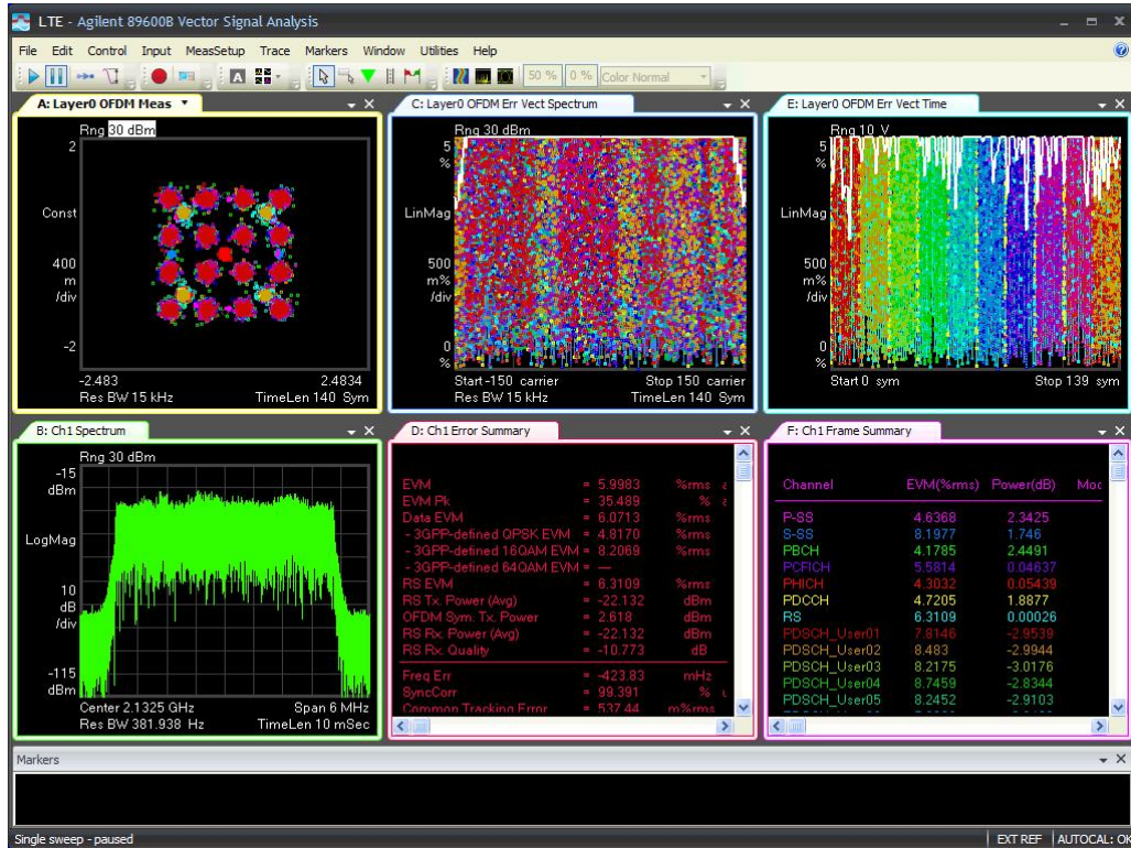
5M-Port 1 -2132.5MHz-TM3.3
