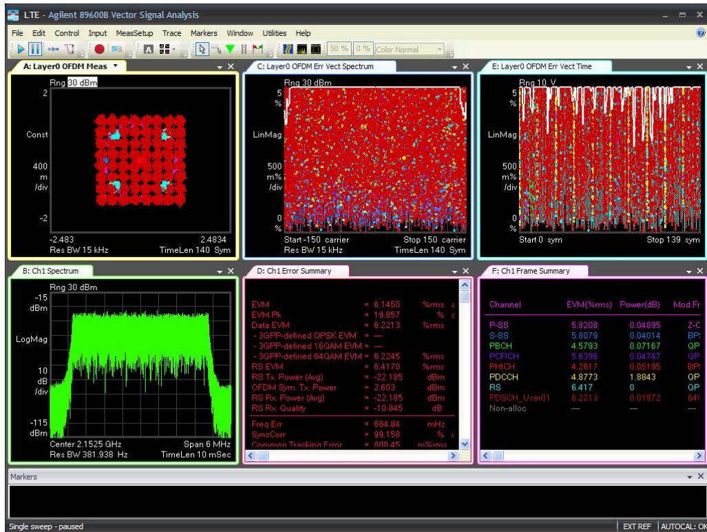
5M-Port 1 - 2152.5MHz-TM3.2
