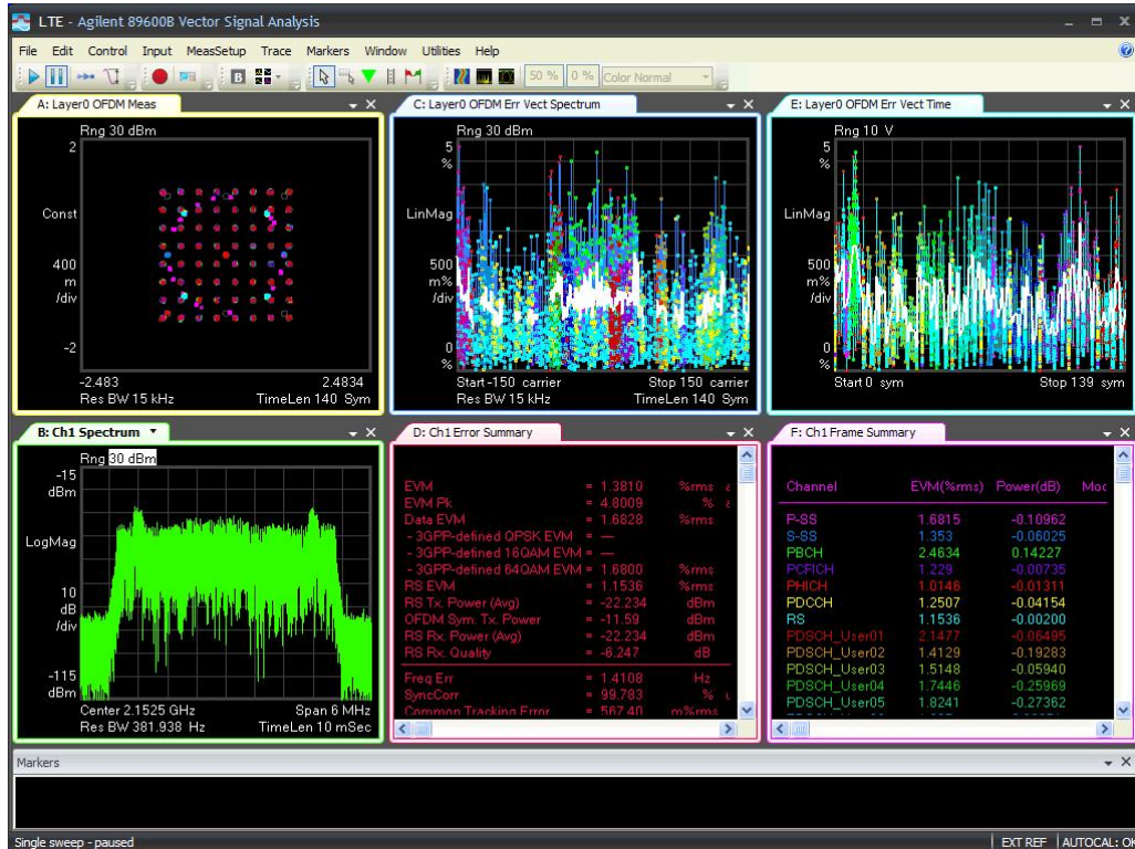
5M-Port 2 -2152.5MHz-TM3.1
