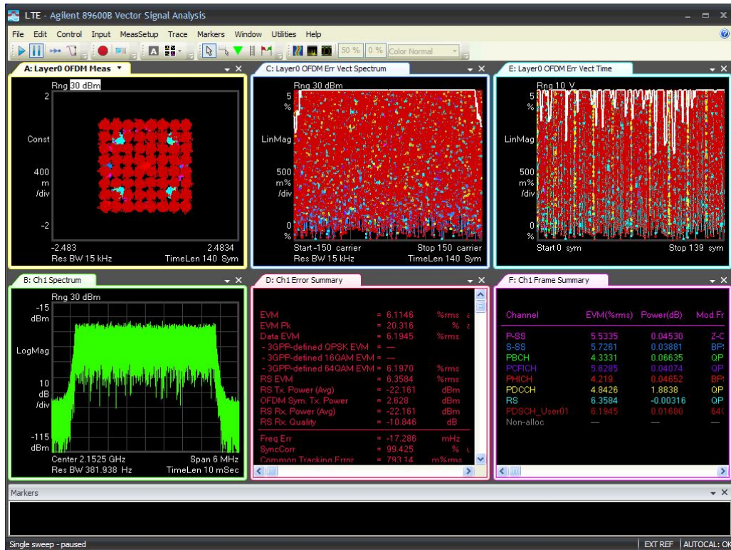
5M-Port 2 -2152.5MHz-TM3.2
