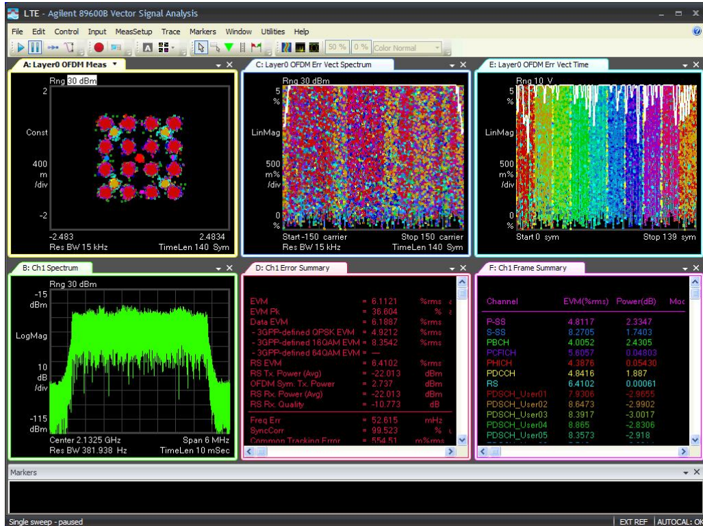
5M-Port 2 -2132.5MHz-TM3.3
