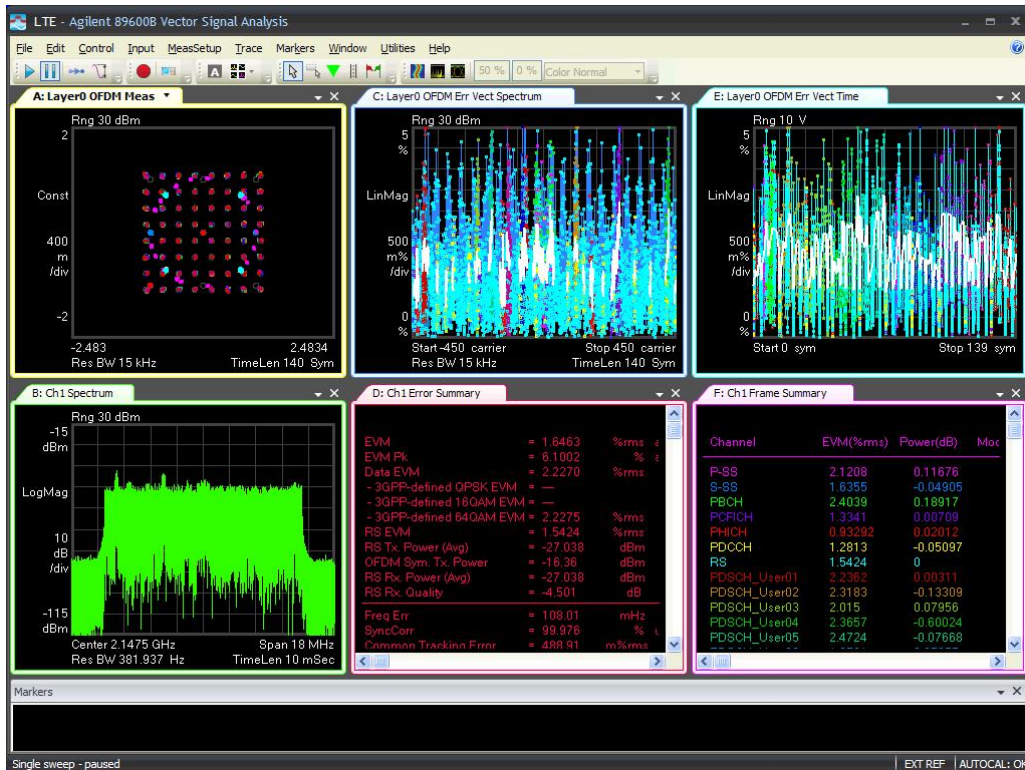
15M-Port 1 -2147.5MHz-TM3.1
