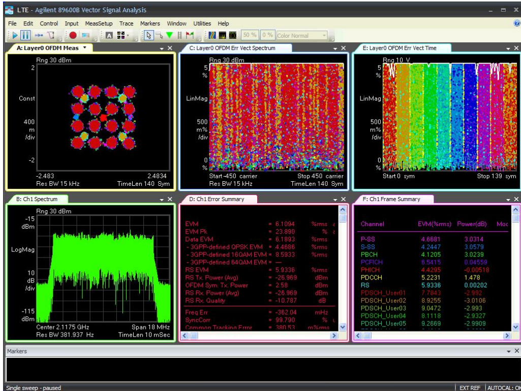
15M-Port 2 -2117.5MHz-TM3.3
