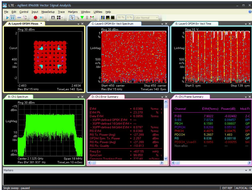
15M-Port 2 -2132.5MHz-TM3.2
