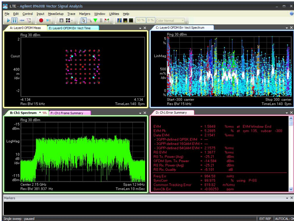
10M-Port 1 -2150MHz-TM3.1
