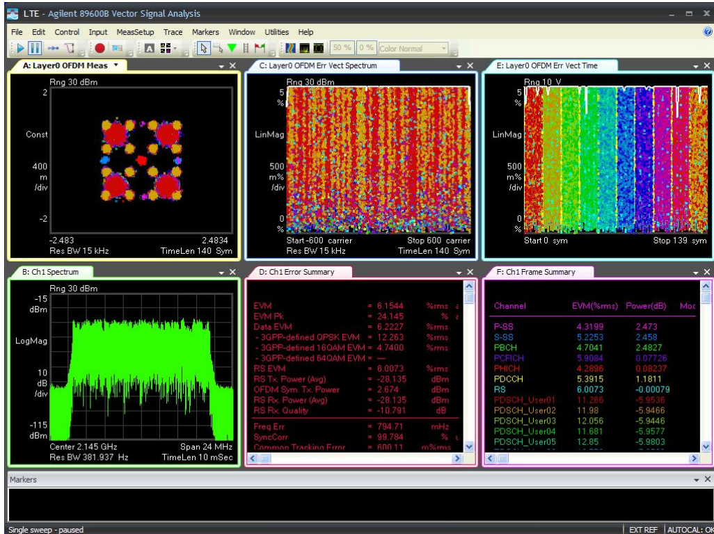
20M-Port 2 -2145MHz-TM3.3
