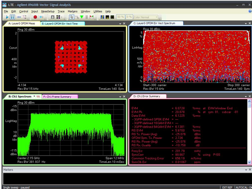
10M-Port 1 -2150MHz-TM3.2
