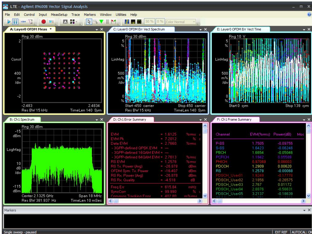
15M-Port 1 -2132.5MHz-TM3.1
