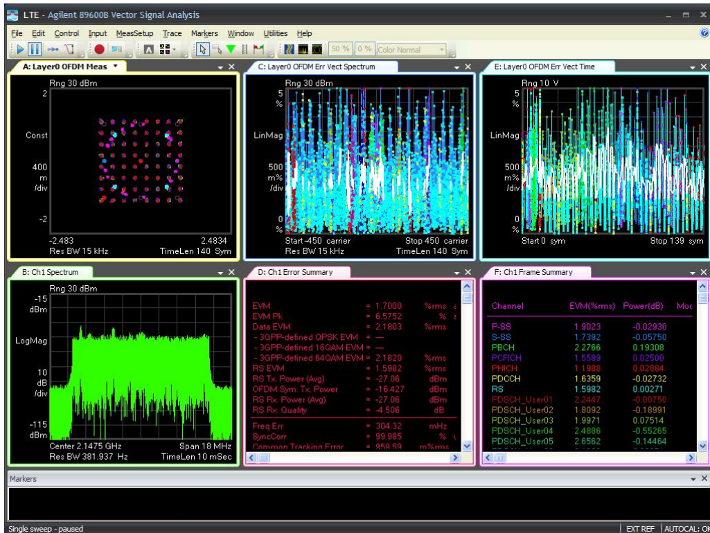
15M-Port 2 -2147.5MHz-TM3.1
