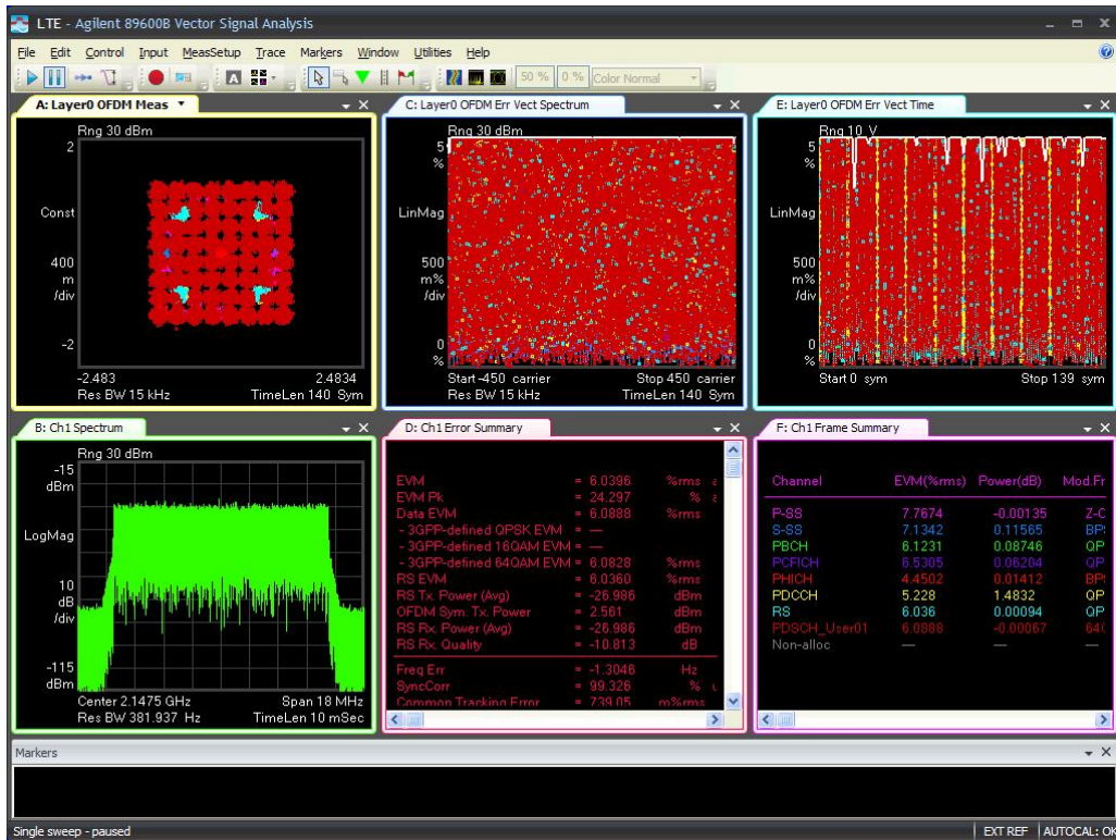
15M-Port 1 -2147.5MHz-TM3.2
