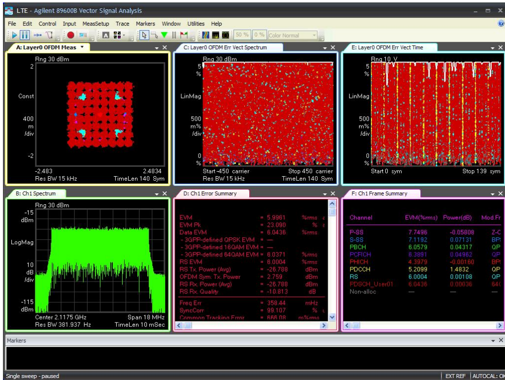
15M-Port 2 -2117.5MHz-TM3.2
