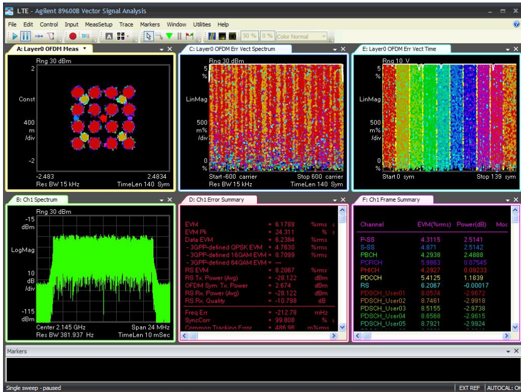
20M-Port 2 -2145MHz-TM3.3
