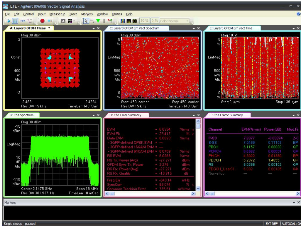
15M-Port 2 -2147.5MHz-TM3.2
