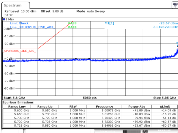
BE-NR-LOW, CHAIN A -DIV1, 802.11n20-HT0, Ch177
