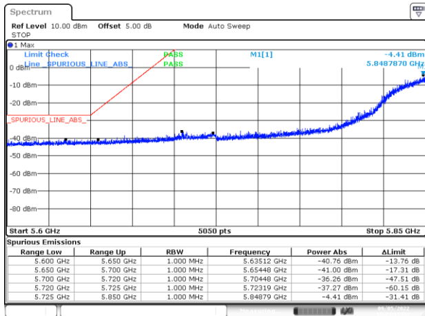
BE-NR-LOW, CHAIN A - DIV2, 802.11ax40-HE0, Ch175
