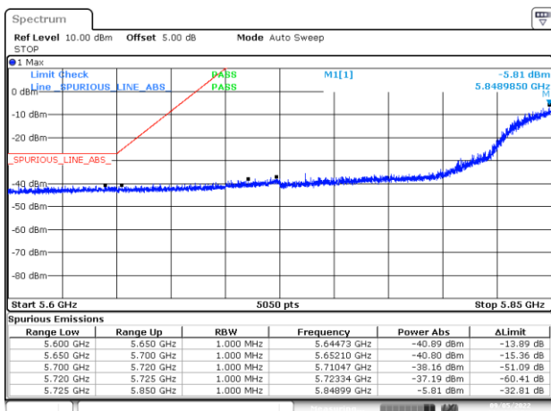
BE-NR-LOW, CHAIN A -DIV1, 802.11n40-HT0, Ch175
