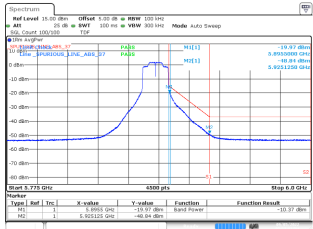
BE-NR-HIGH, CHAIN A - DIV2, 802.11ax20-HE0, Ch177
