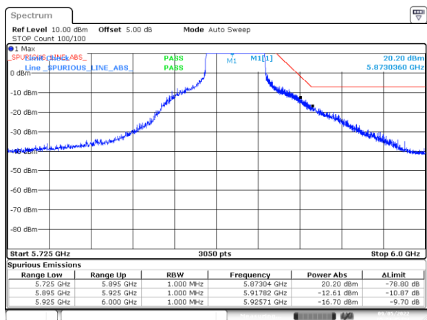
BE-NR-HIGH, CHAIN A - DIV2, 802.11ax40-HE0, Ch175
