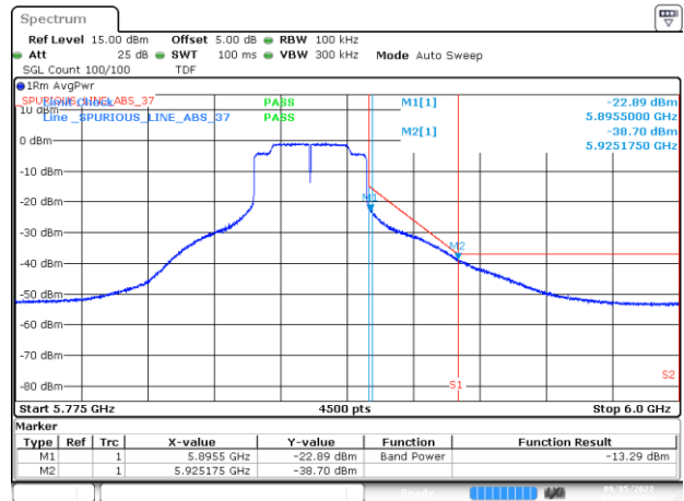
BE-NR-HIGH, CHAIN A - DIV2, 802.11ax40-HE0, Ch175
