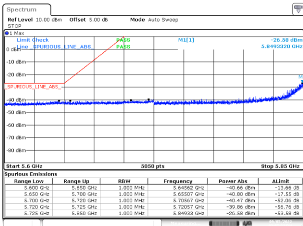
BE-NR-LOW, CHAIN A -DIV1, 802.11a20-6Mbps, Ch177
