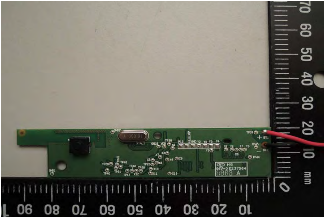
2.4G Antenna
