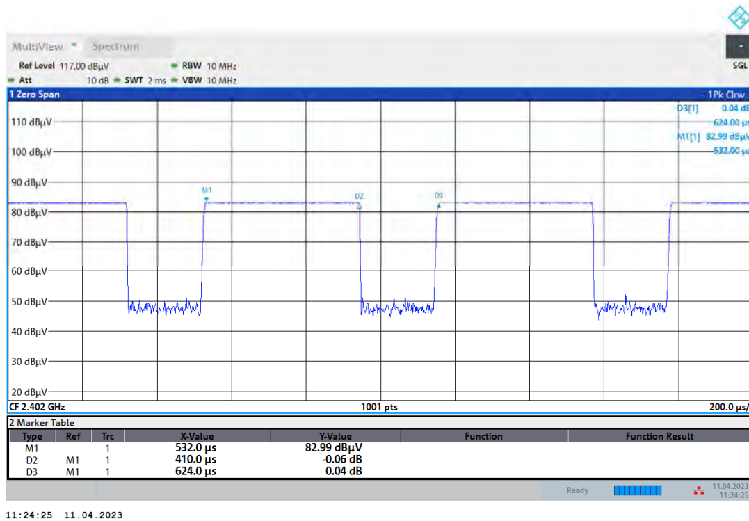
BLE 1 Mbps
