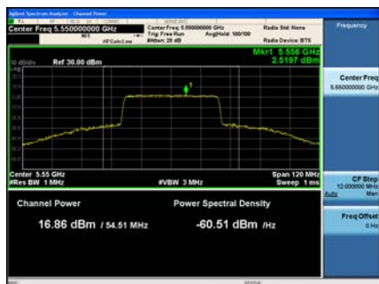
Antenna A
