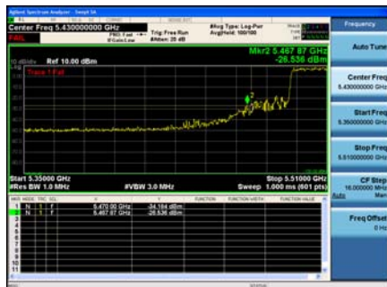
Antenna A
