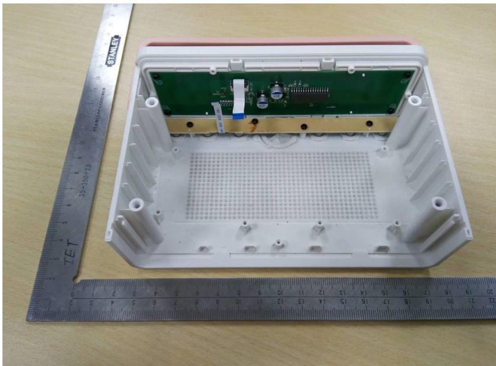
(12) EUT Photo
