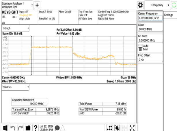
802.11ax_40MHz_Chain1_6925MHz_RU242_61
