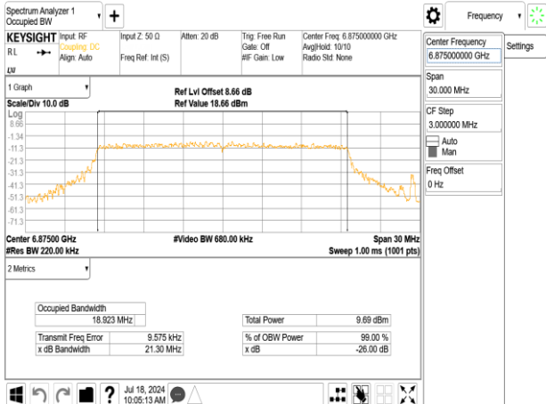
802.11ax_20MHz_Chain1_6875MHz
