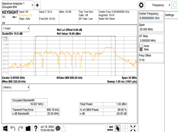
802.11ax_20MHz_Chain1_6855MHz_RU52_40
