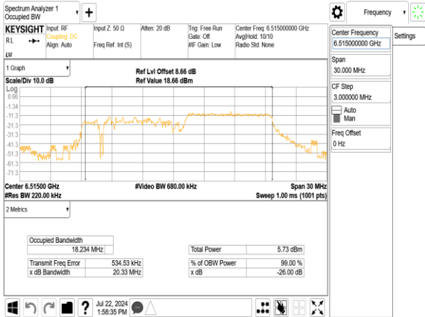
802.11ax_20MHz_Chain1_6515MHz_RU106_54
