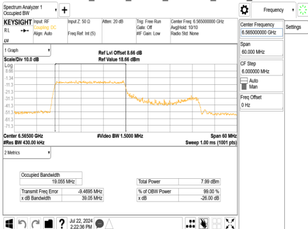
802.11ax_40MHz_Chain1_6565MHz_RU242_61
