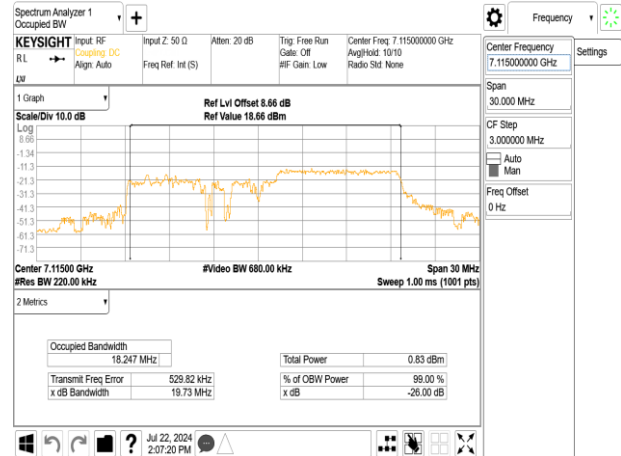
802.11ax_20MHz_Chain1_7115MHz_RU26_8
