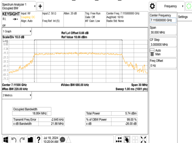
802.11ax_20MHz_Chain1_7115MHz
