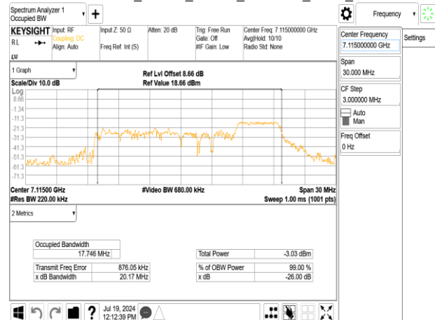
802.11ax_20MHz_Chain1_7115MHz_RU52_40
