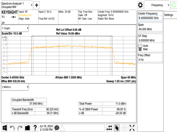
802.11ax_40MHz_Chain1_6405MHz_RU242_62
