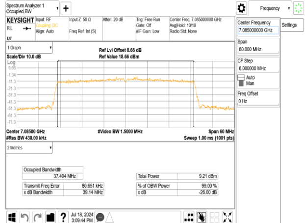
802.11ax_40MHz_Chain1_7085MHz_RU242_62
