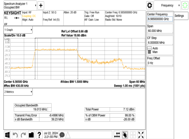
802.11ax_40MHz_Chain0_6565MHz_RU242_61
