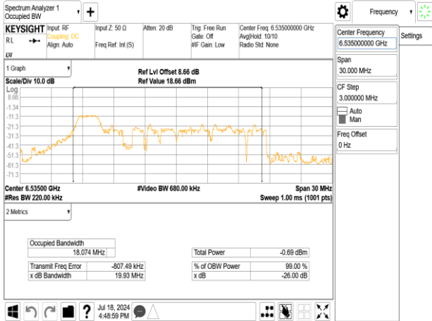
802.11ax_20MHz_Chain1_6535MHz_RU52_37
