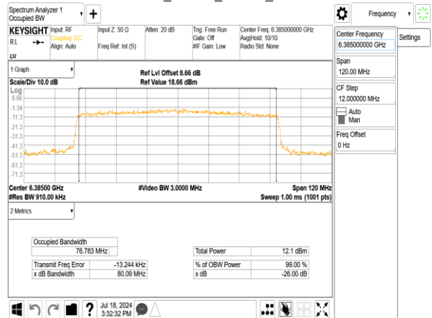
802.11ax_80MHz_Chain0_6385MHz_RU484_66
