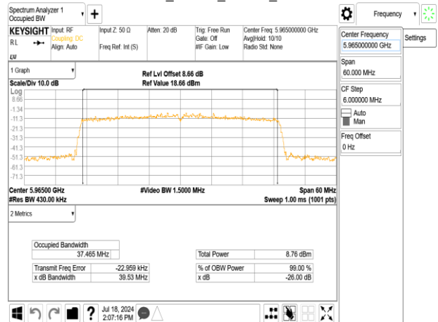
802.11ax_40MHz_Chain1_5965MHz_RU242_61
