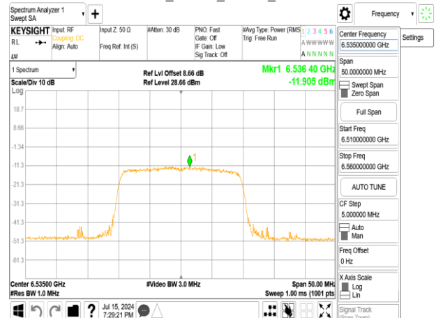
802.11ax_20MHz_Chain1_6535MHz
