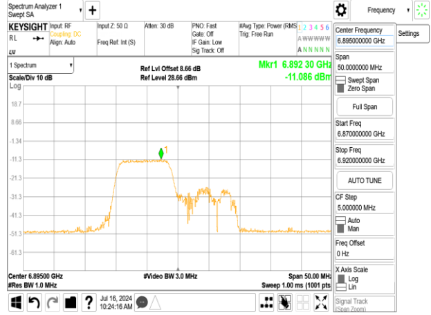
802.11ax_20MHz_Chain1_6895MHz_RU26_0
