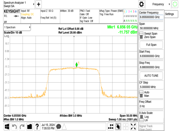
802.11ax_20MHz_Chain1_6855MHz_RU106_54
