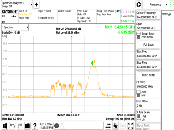
802.11ax_20MHz_Chain1_6415MHz_RU52_40
