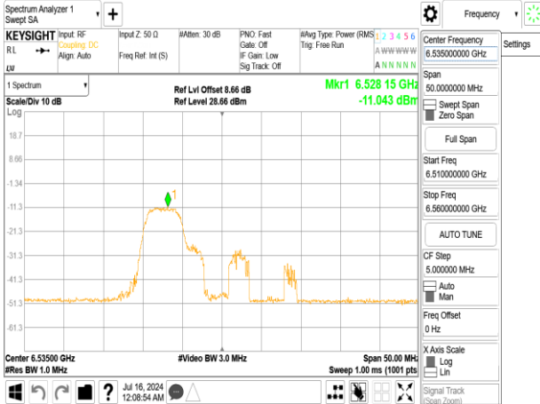
802.11ax_20MHz_Chain1_6535MHz_RU52_37
