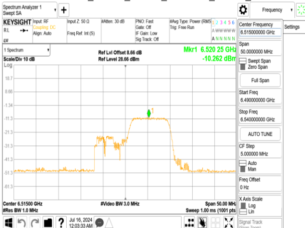
802.11ax_20MHz_Chain1_6515MHz_RU106_54
