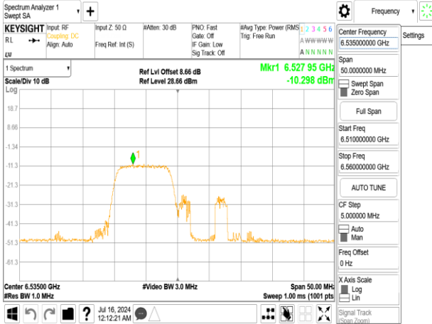
802.11ax_20MHz_Chain1_6535MHz_RU26_0
