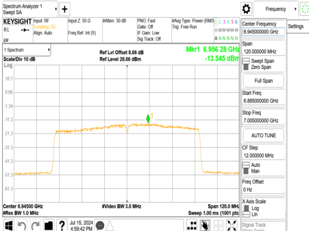
802.11ac_80MHz_Chain1_6945MHz
