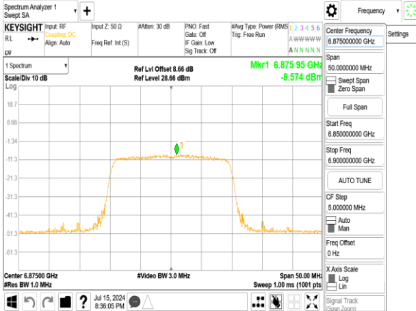
802.11ax_20MHz_Chain1_6875MHz
