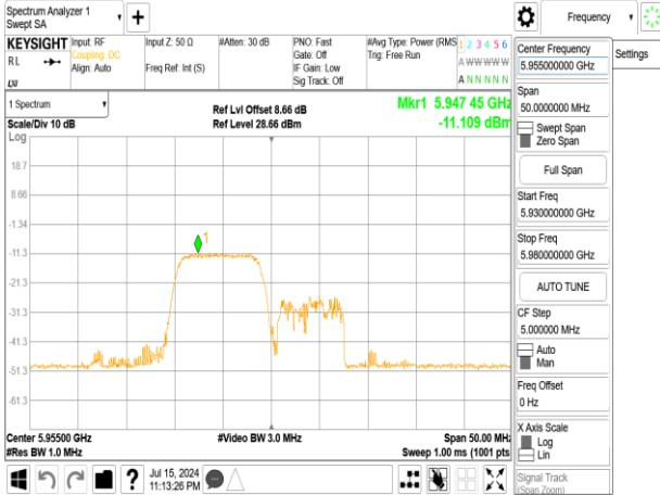
802.11ax_20MHz_Chain1_5955MHz_RU26_0
