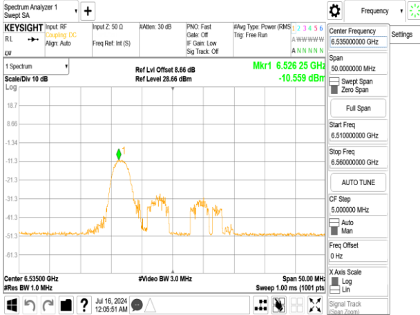
802.11ax_20MHz_Chain0_6535MHz_RU52_37
