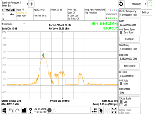
802.11ax_20MHz_Chain0_5955MHz_RU52_37
