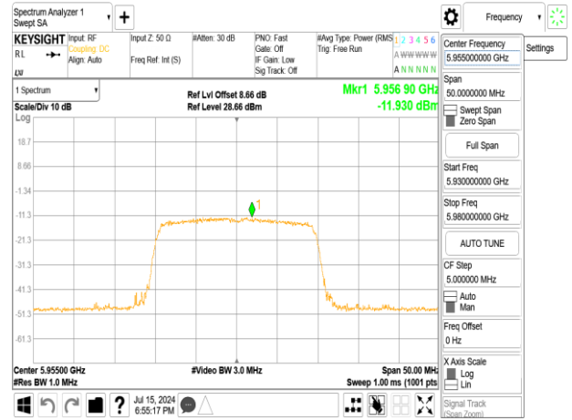
802.11ax_20MHz_Chain1_5955MHz
