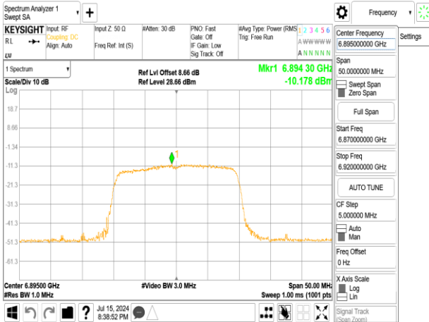
802.11ax_20MHz_Chain0_6895MHz
