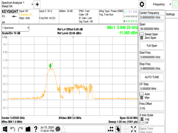
802.11ax_20MHz_Chain1_5955MHz_RU52_37
