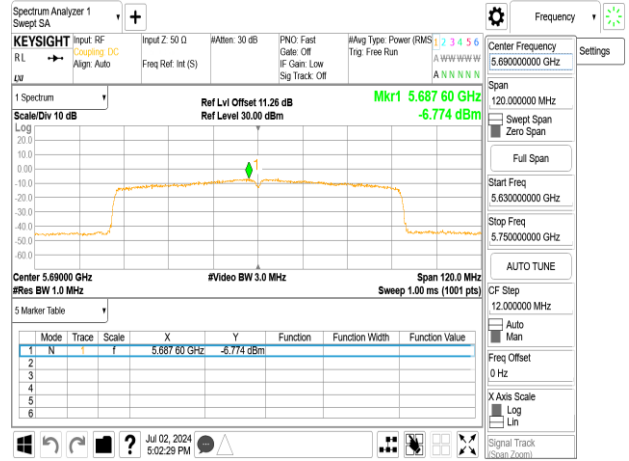
802.11ac_80MHz_Chain1_5690MHz_UNII 3
