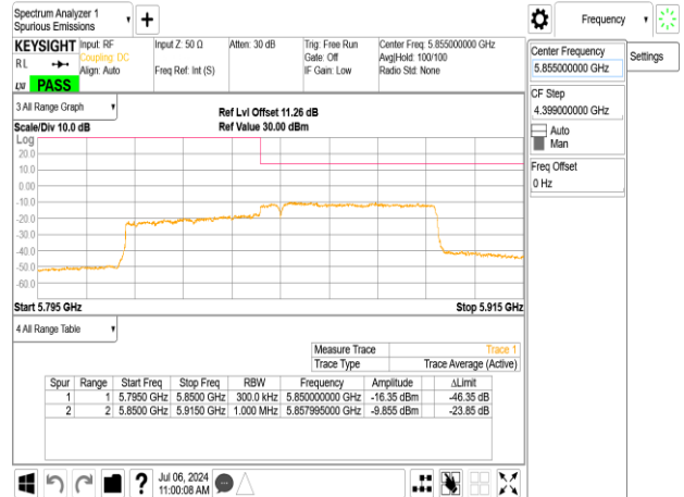
802.11ac_80MHz_Chain0_5855MHz_UNII 2C
