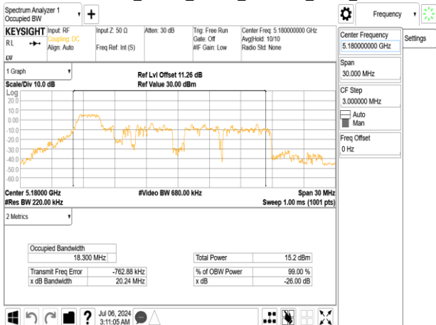
802.11ax_20MHz_Chain0_5180MHz_RU26_0
