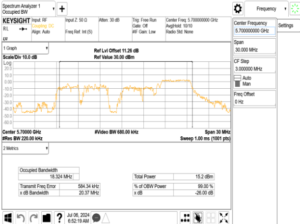
802.11ax_20MHz_Chain0_5700MHz_RU52_40
