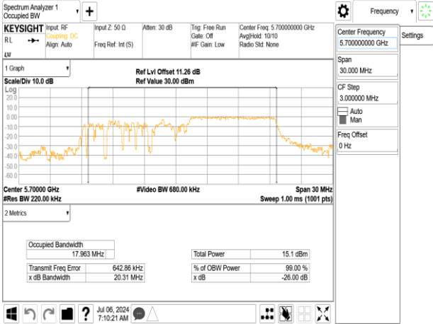
802.11ax_20MHz_Chain0_5700MHz_RU26_8
