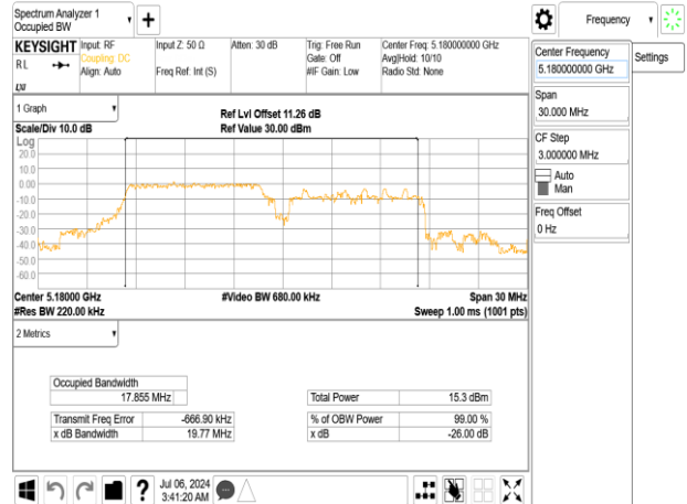
802.11ax_20MHz_Chain1_5180MHz_RU106_53
