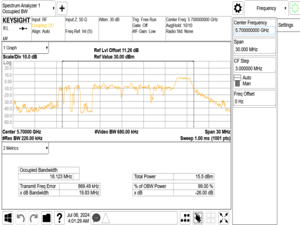
802.11ax_20MHz_Chain0_5700MHz_RU52_40
