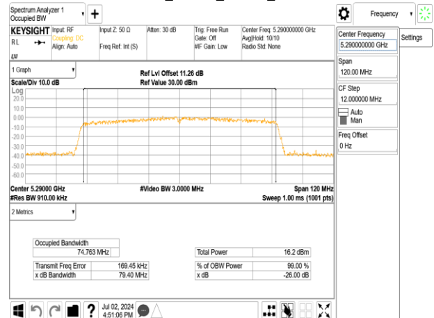
802.11ac_80MHz_Chain0_5290MHz
