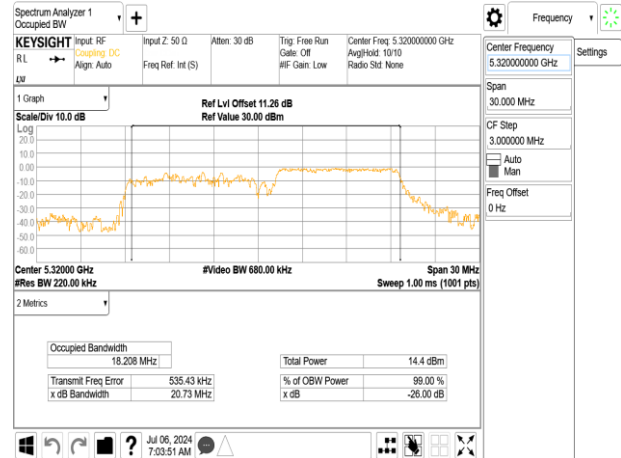
802.11ax_20MHz_Chain0_5320MHz_RU26_8
