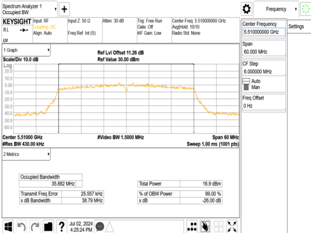
802.11n_40MHz_Chain1_5510MHz
