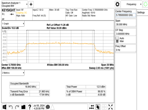
802.11ax_20MHz_Chain0_5785MHz
