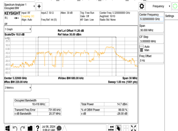
802.11ax_20MHz_Chain0_5320MHz_RU52_40
