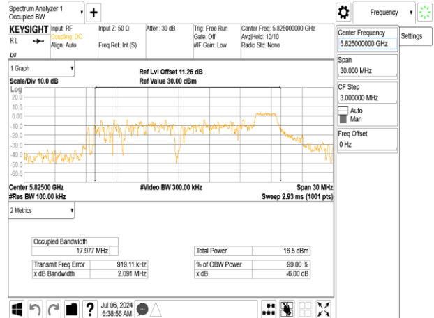
802.11ax_20MHz_Chain0_5825MHz_RU26_8
