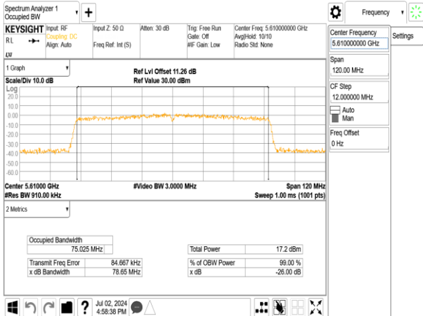
802.11ac_80MHz_Chain1_5610MHz
