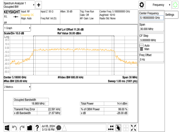
802.11ax_20MHz_Chain1_5180MHz_RU106_53
