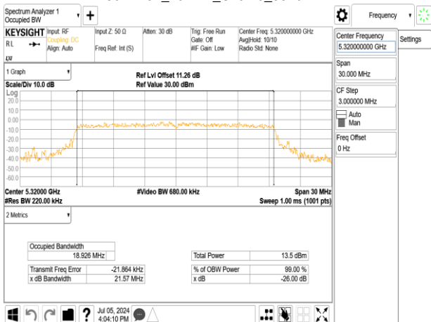
802.11ax_20MHz_Chain0_5320MHz
