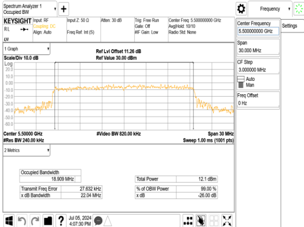
802.11ax_20MHz_Chain0_5500MHz_RU106_53
