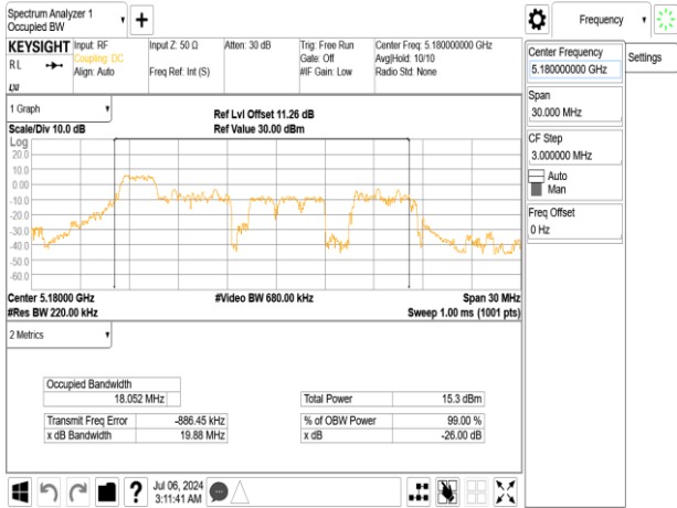
802.11ax_20MHz_Chain1_5180MHz_RU52_37
