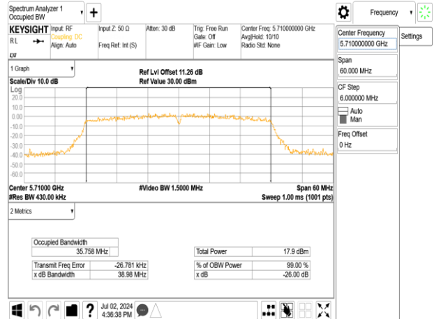
802.11n_40MHz_Chain1_5710MHz
