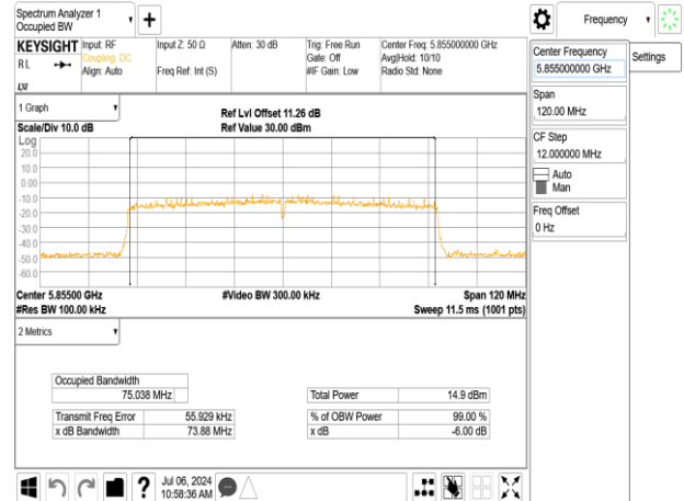
802.11ac_80MHz_Chain1_5855MHz
