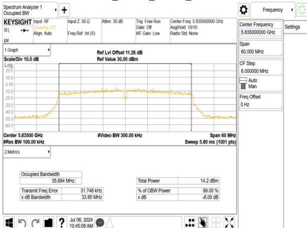
802.11n_40MHz_Chain1_5835MHz
