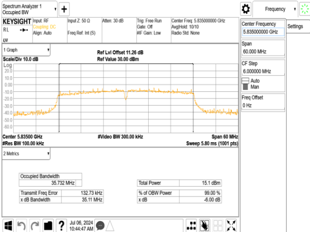
802.11n_40MHz_Chain0_5835MHz
