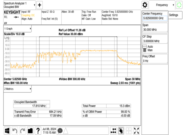
802.11ax_20MHz_Chain0_5825MHz_RU26_8
