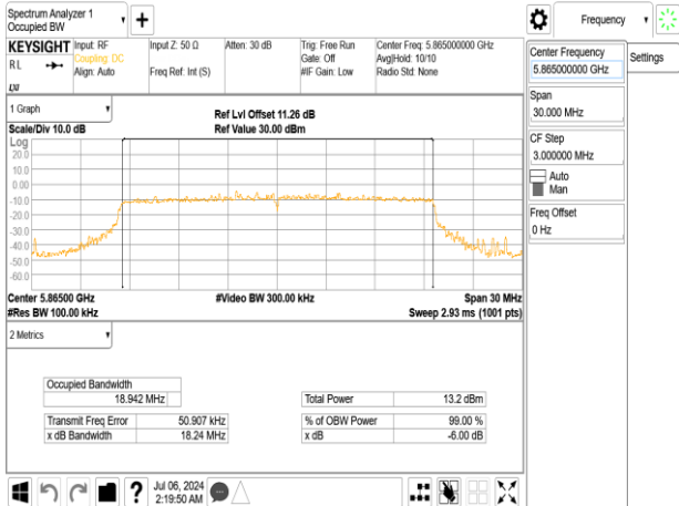
802.11ax_20MHz_Chain0_5865MHz
