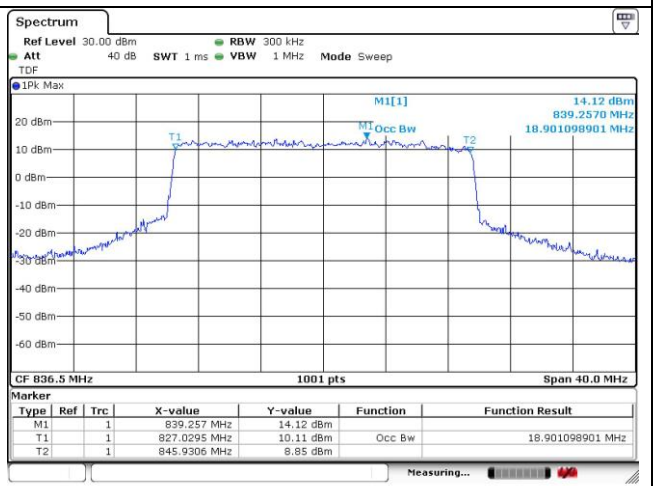
20 MHz CP-OFDM QPSK
