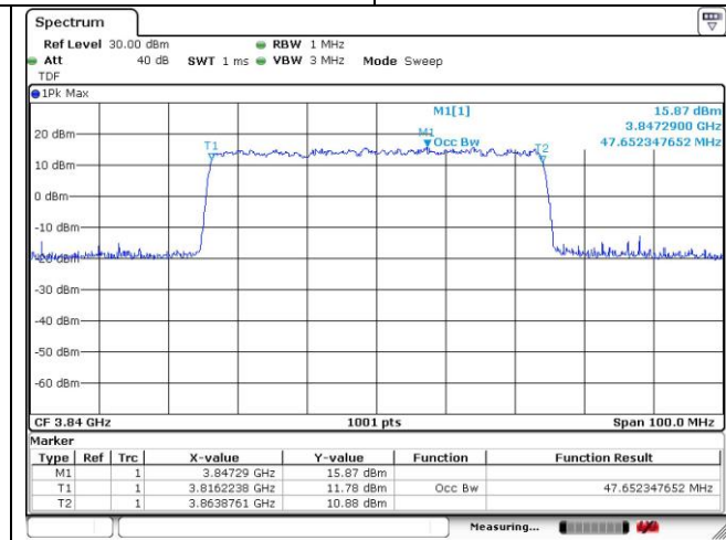
50 MHz CP-OFDM 16QAM
