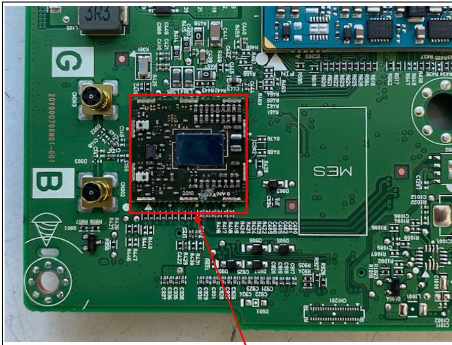
BT/WIFI Module
