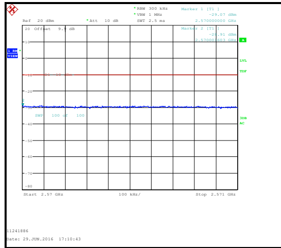
QPSK / Upper Band Edge
