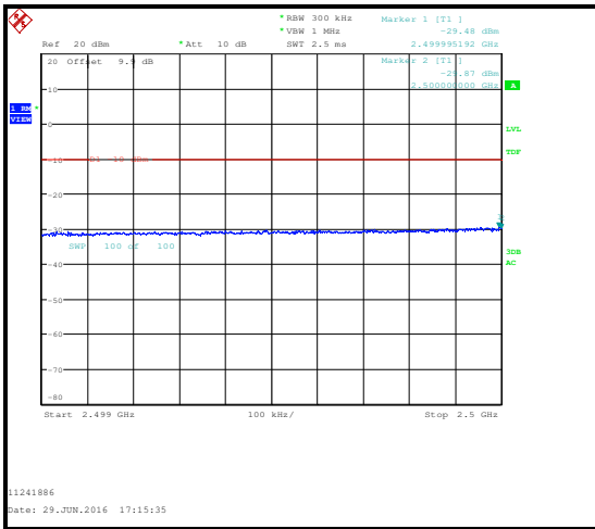
QPSK / Lower Band Edge
