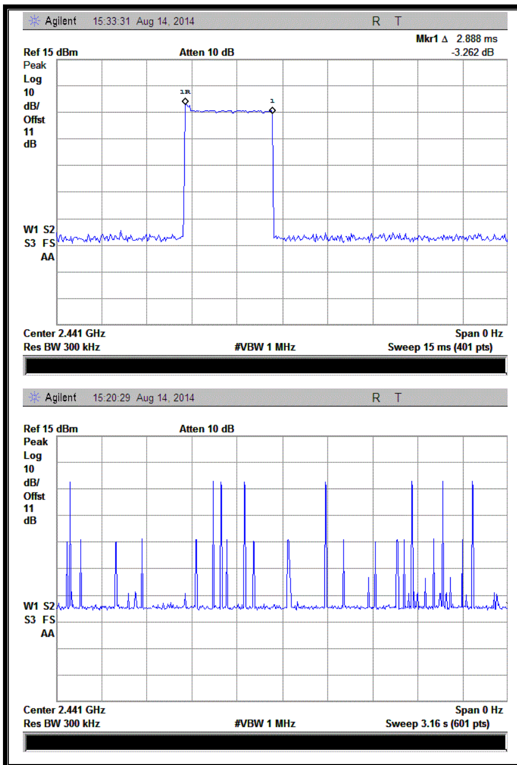
(Plot C: DH5 @ \pi/4 -DQPSK)
