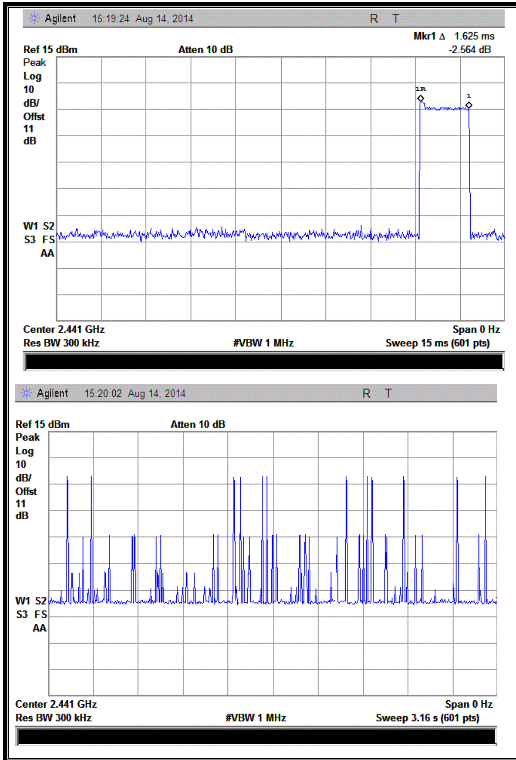
(Plot B: DH3 @ \pi/4 -DQPSK)
