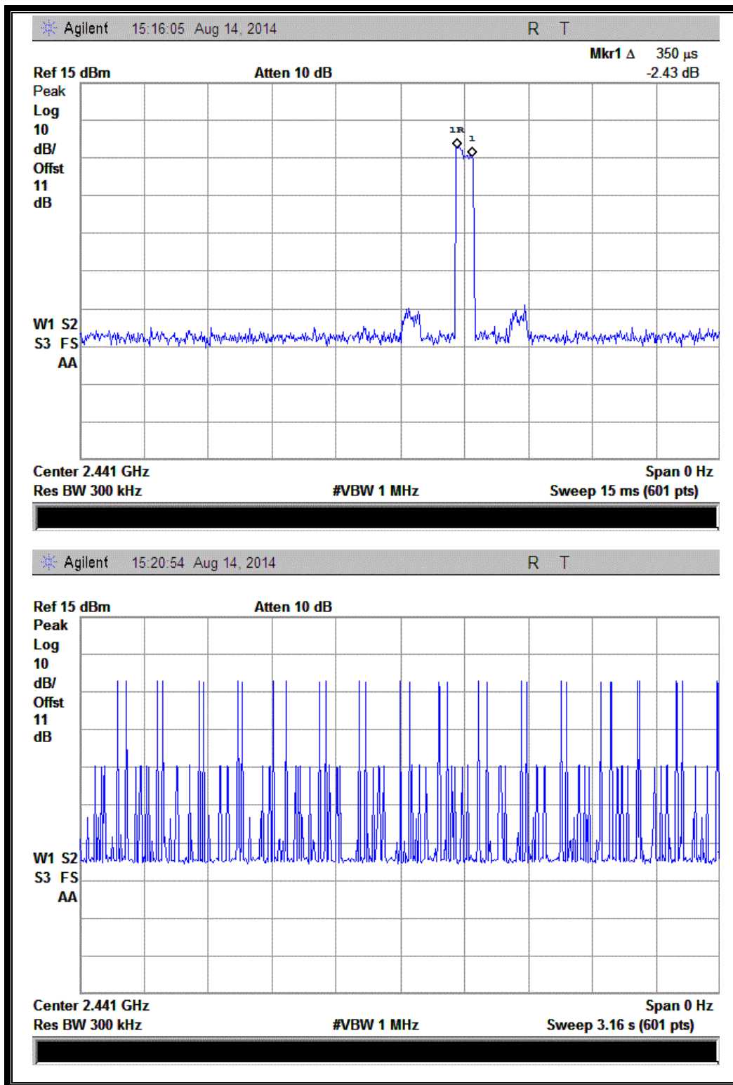
(Plot A: DH1 @ \pi/4 -DQPSK)
