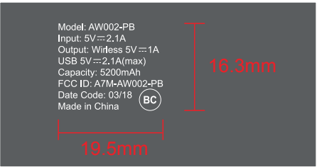
产品底面丝印 颜色：白色
