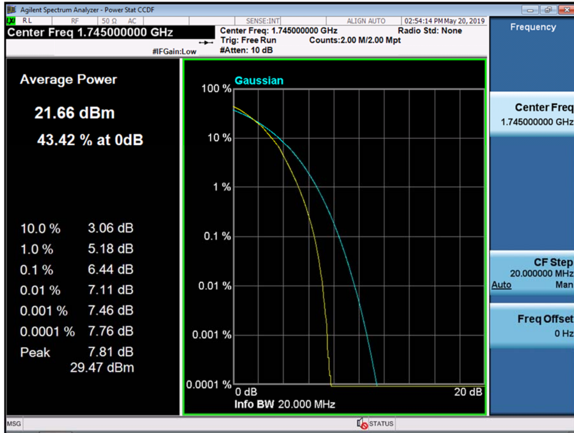
BAND 66/4. PAR Plot (20M BW_Ch.132322_64QAM_RB100_0)
