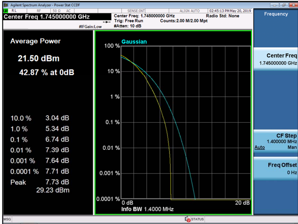
BAND 66/4. PAR Plot (1.4M BW_Ch.132322_64QAM_RB6_0)
