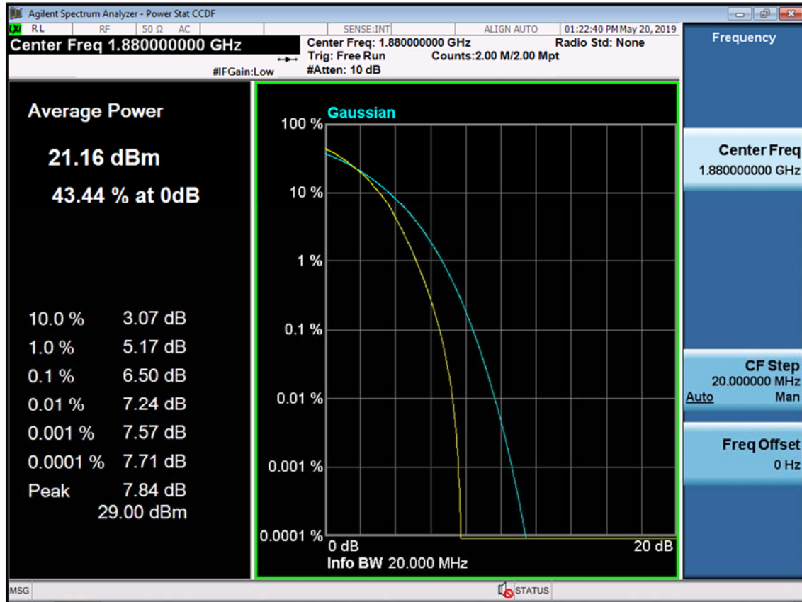
BAND 2. PAR Plot (20M BW Ch.18900 64QAM RB 100_0)
