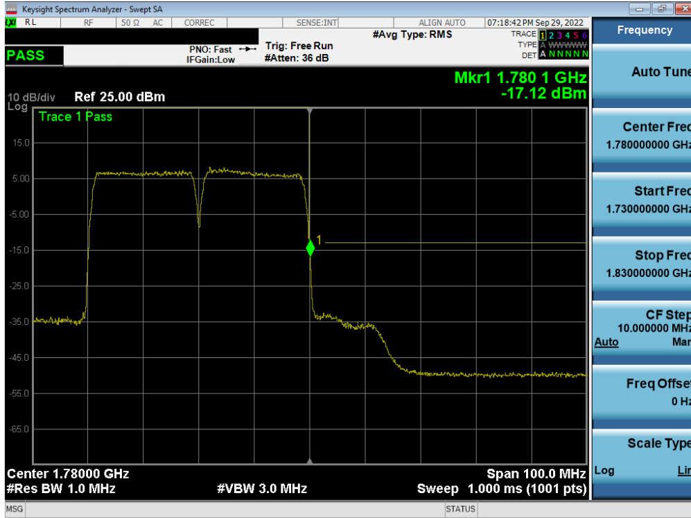
Plot 7-321. Upper Band Edge Plot (ULCA LTE Band 66 - ANT A)
