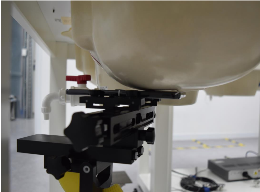
Left Touch
