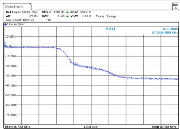
UNII-3 / 802.11a
