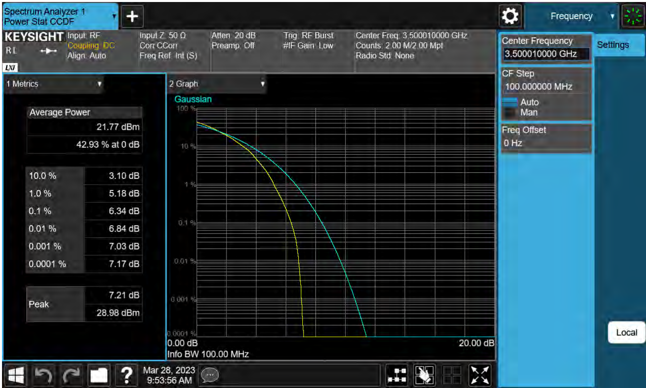
Sub6 n77. PAR Plot (100 M BW_Ch.633334_64QAM)
