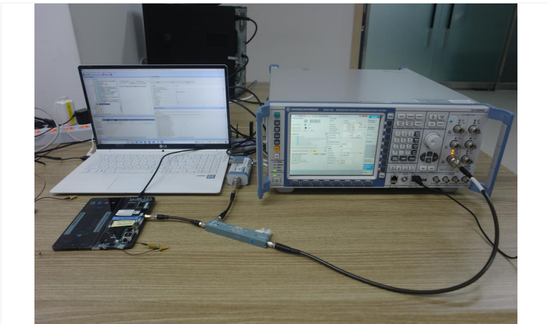
Test setup photo- (7-1 (d) WLAN)
