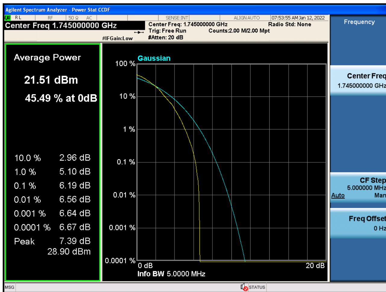
Sub6 n66. PAR Plot (5 M BW_Ch.349000_64QAM_Full RB)
