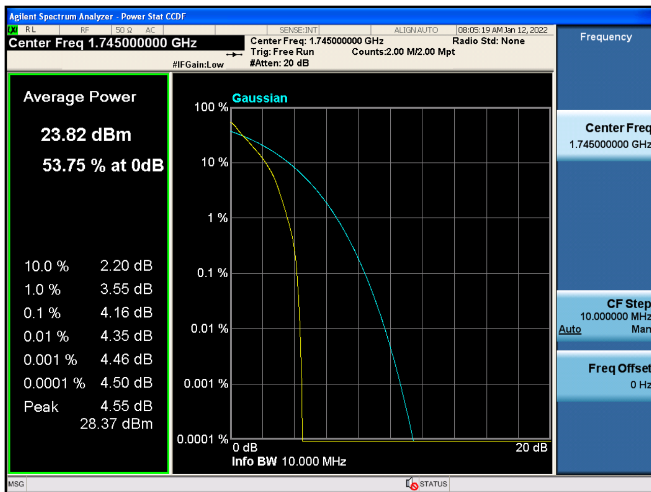
Sub6 n66. PAR Plot (10 M BW_Ch.349000_ BPSK_ Full RB)
