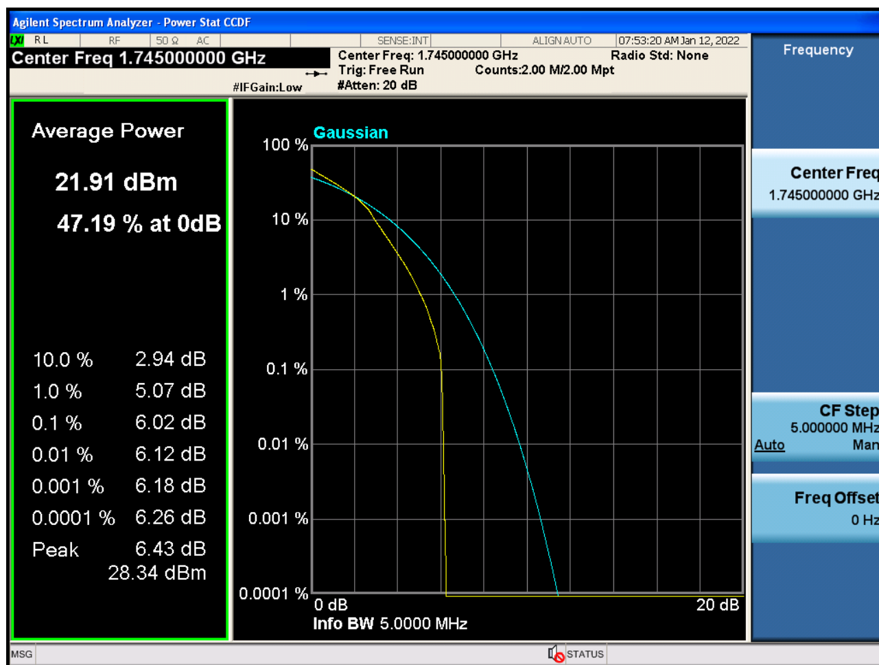
Sub6 n66. PAR Plot (5 M BW_Ch.349000_16QAM_Full RB)
