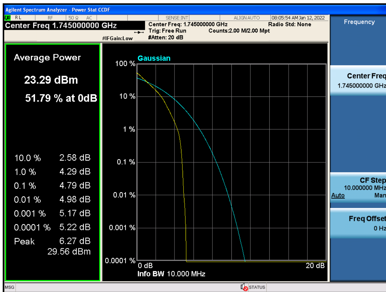
Sub6 n66. PAR Plot (10 M BW_Ch.349000_QPSK_Full RB)
