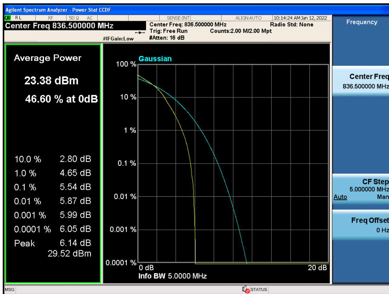
Sub6 n5. PAR Plot (5 M BW_Ch. 167300_16QAM_Full RB_0)
