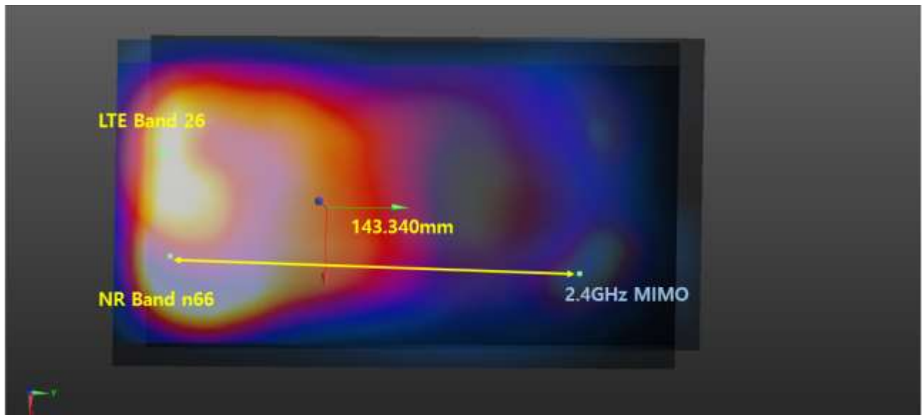
Plot #10 NR Band n66+ LTE Band 26+ 2.4 GHz WLAN MIMO
