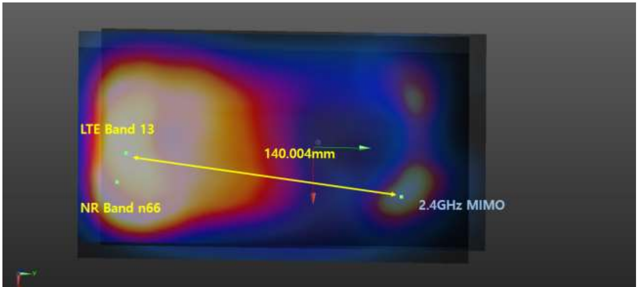
Plot #9 NR Band n66+ LTE Band 13+ 2.4 GHz WLAN MIMO
